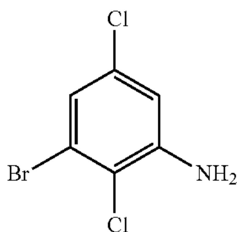
3-bromo-2,5-dichloroaniline
