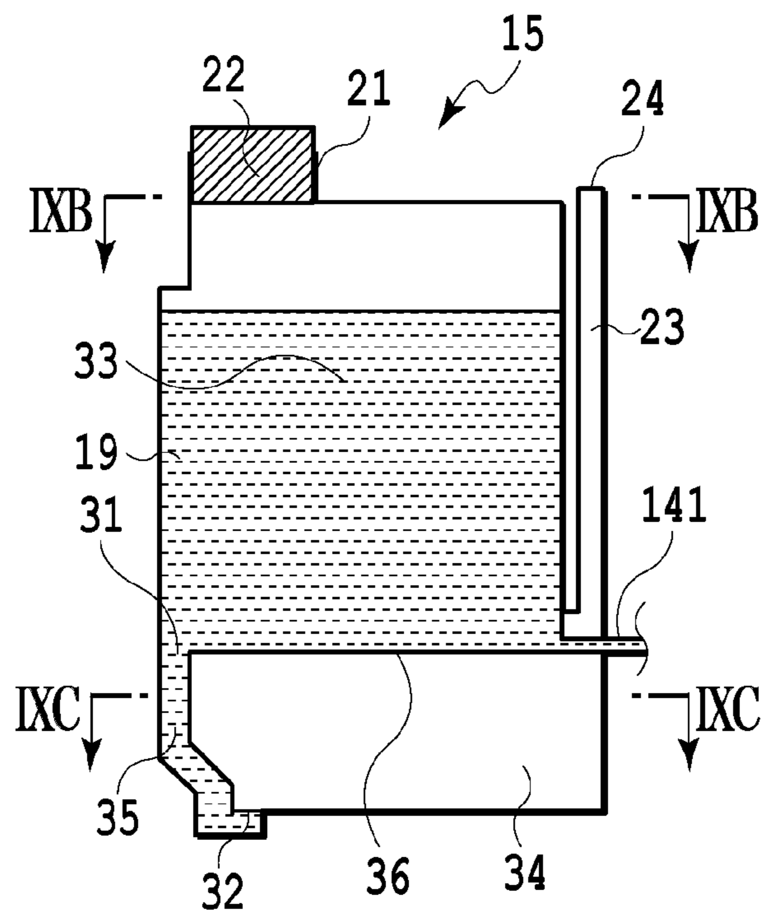
FIG. 9A
