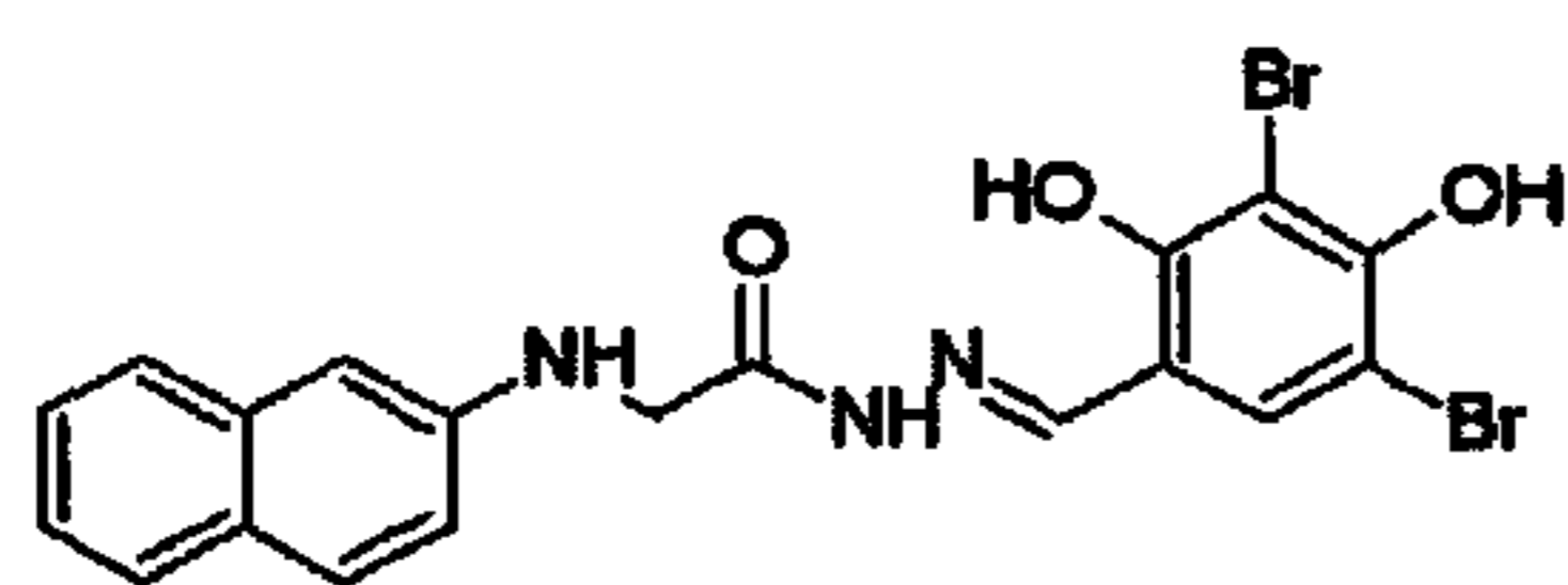
GlyH-101
