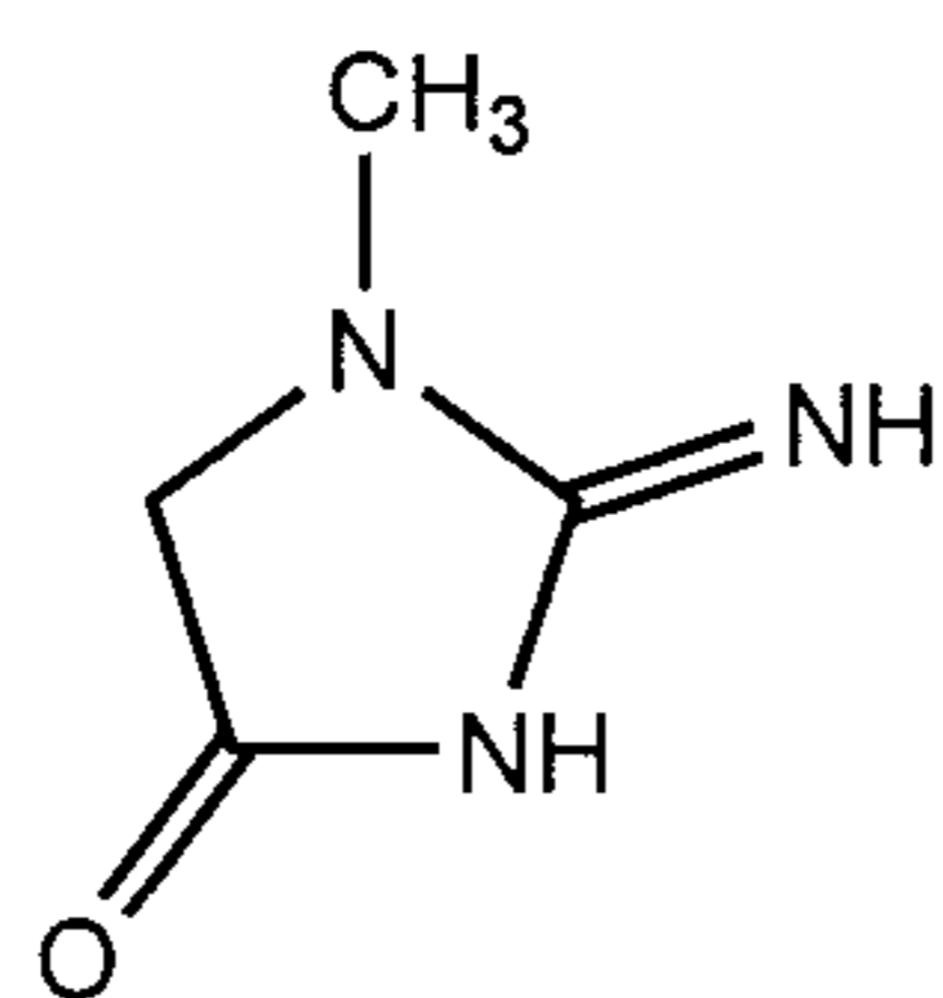
Creatinine (1) MW: 113
