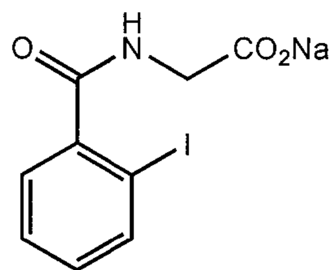
o-Iodohippurate (2) MW: 327
