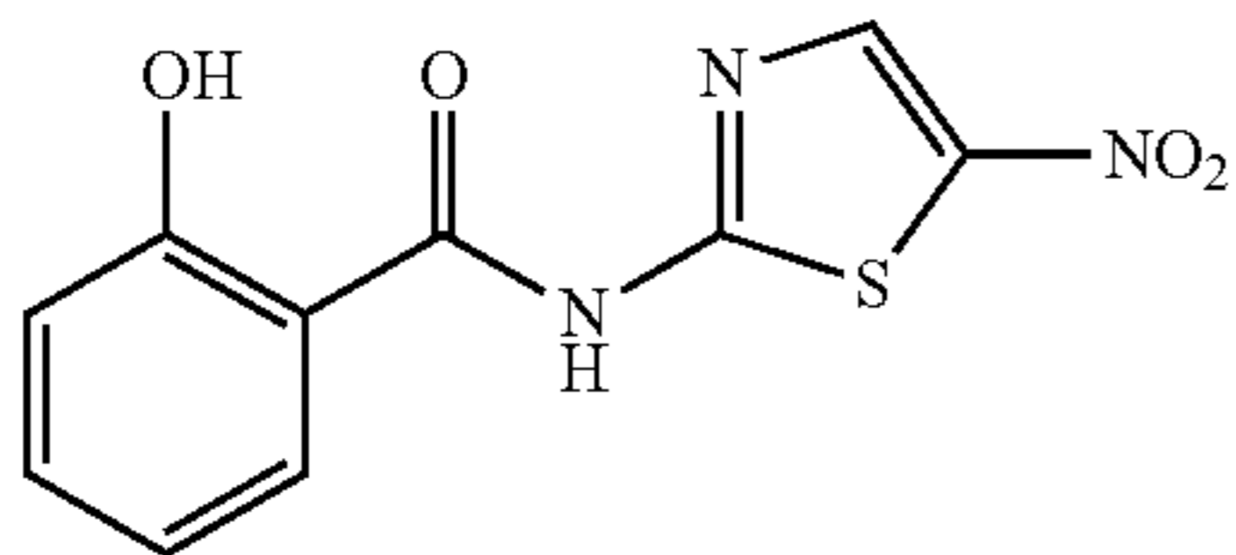
Tizoxanide
