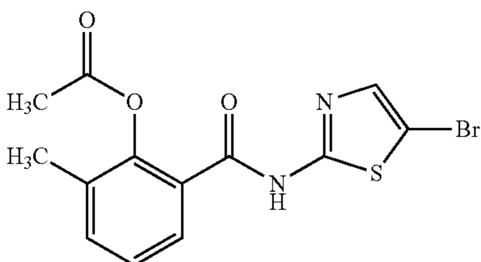
Tizoxanide
