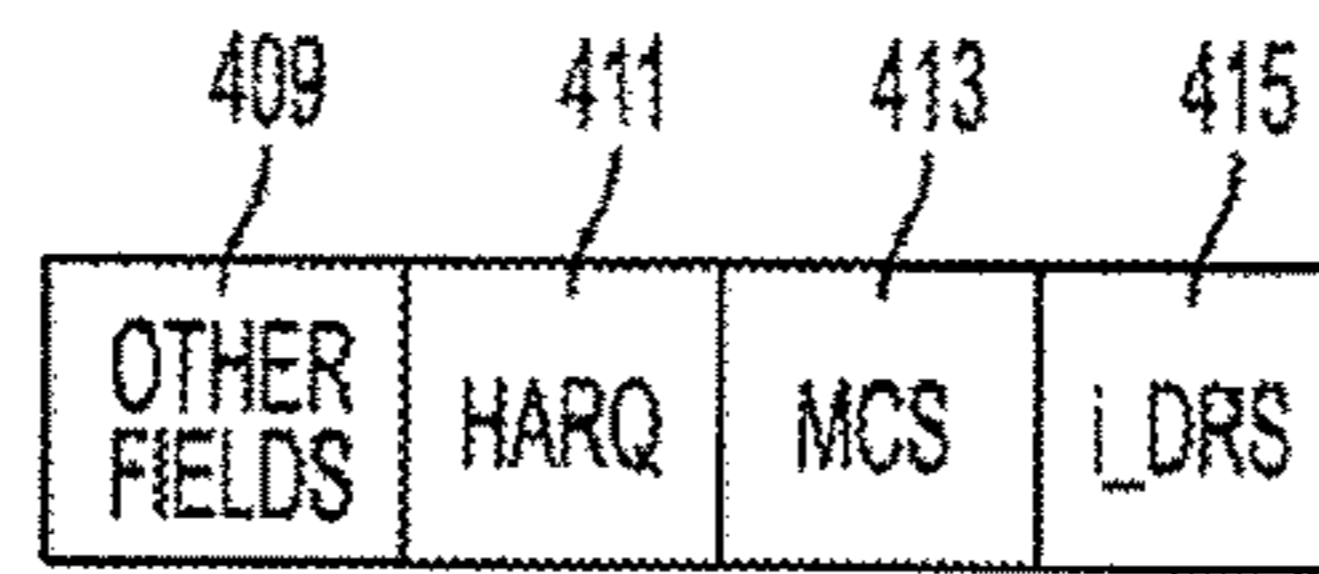
DCI FORMAT 1E FIG. 4B RELATED ART
