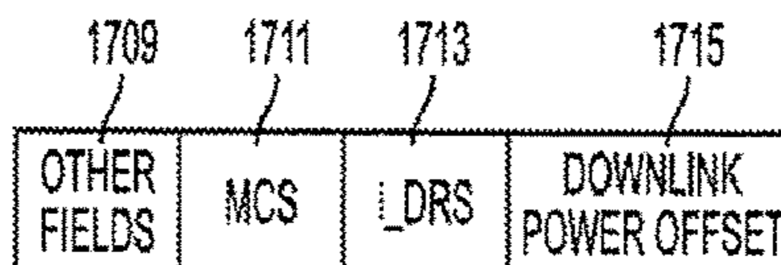
DCI FORMAT 1F_b FIG. 17B
