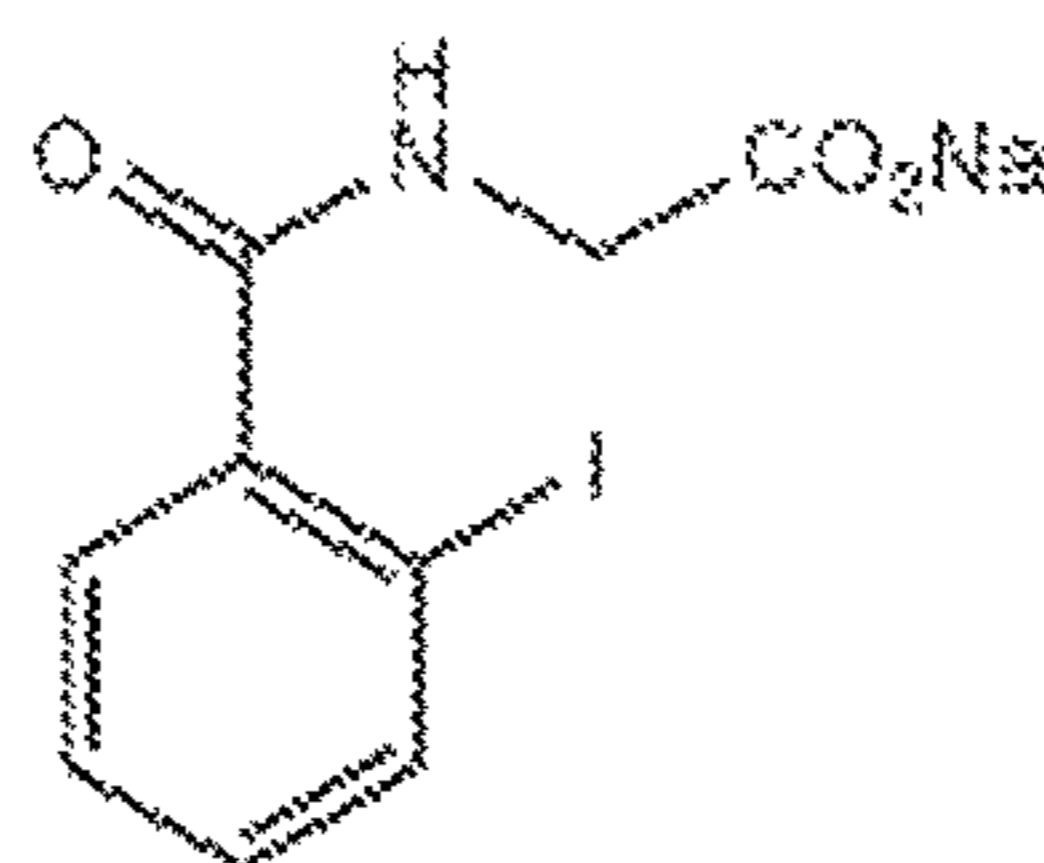
o-Iodohippurate (2) MW: 327
