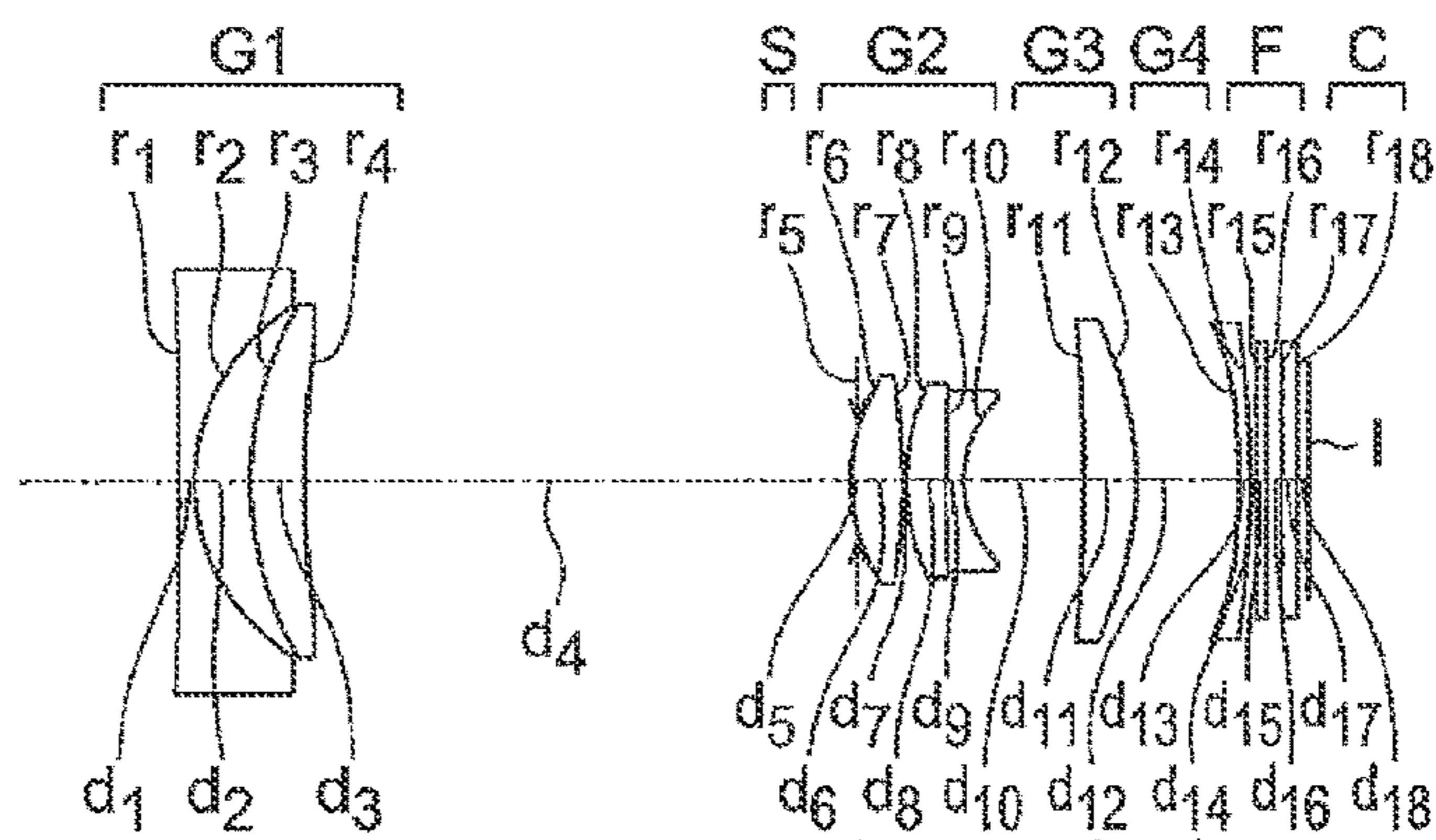
FIG. 3A
