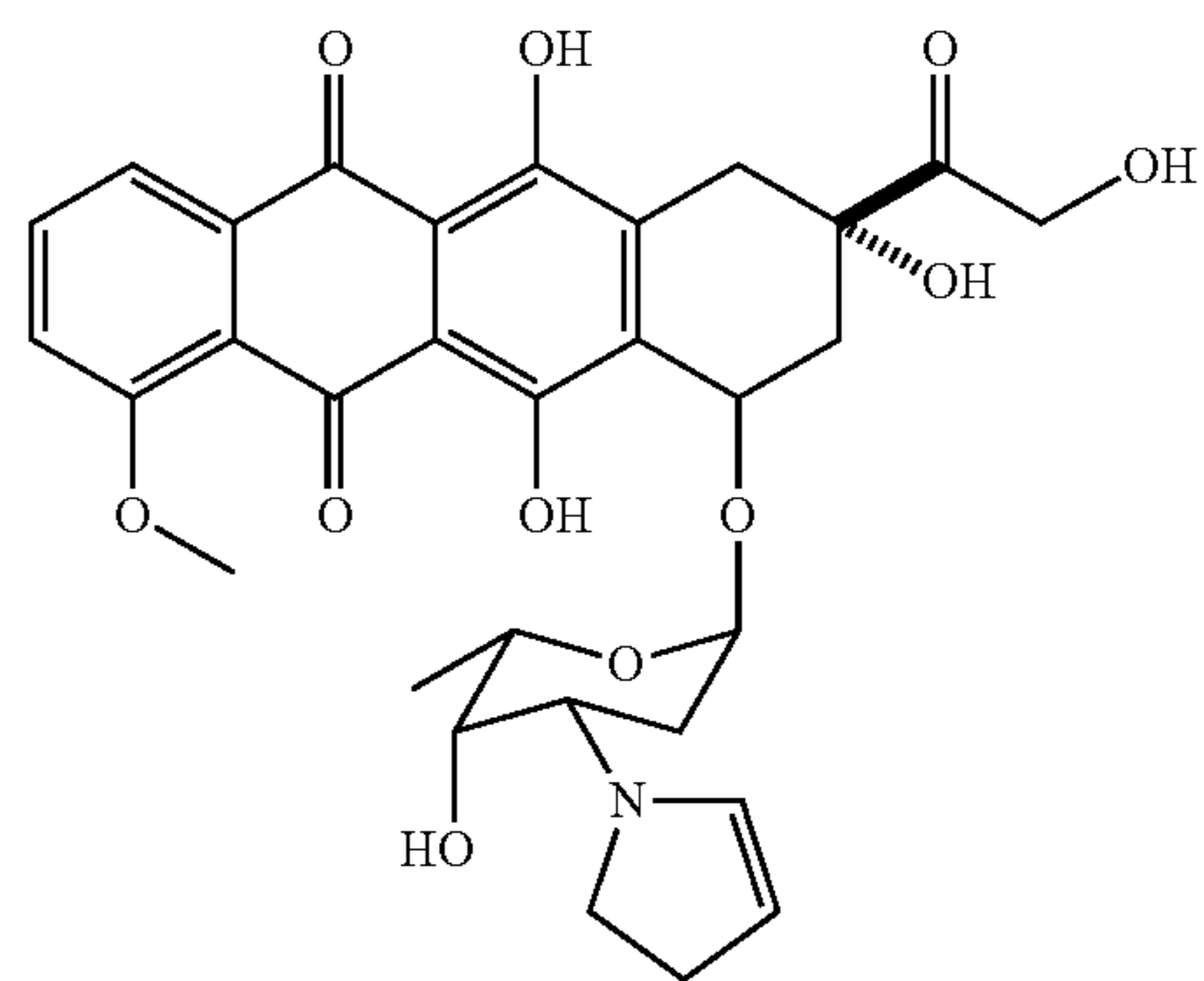
2-Pyrrolinodoxorubicin (4)
