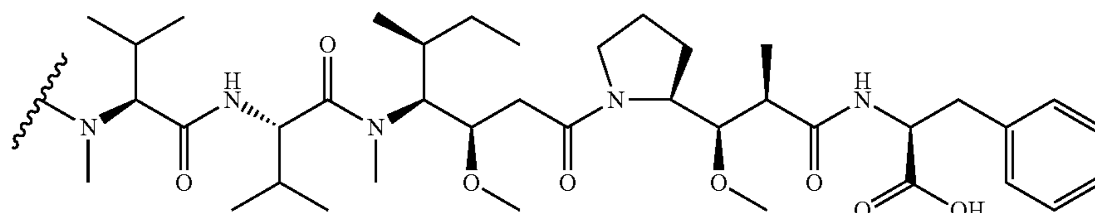
MMAF
