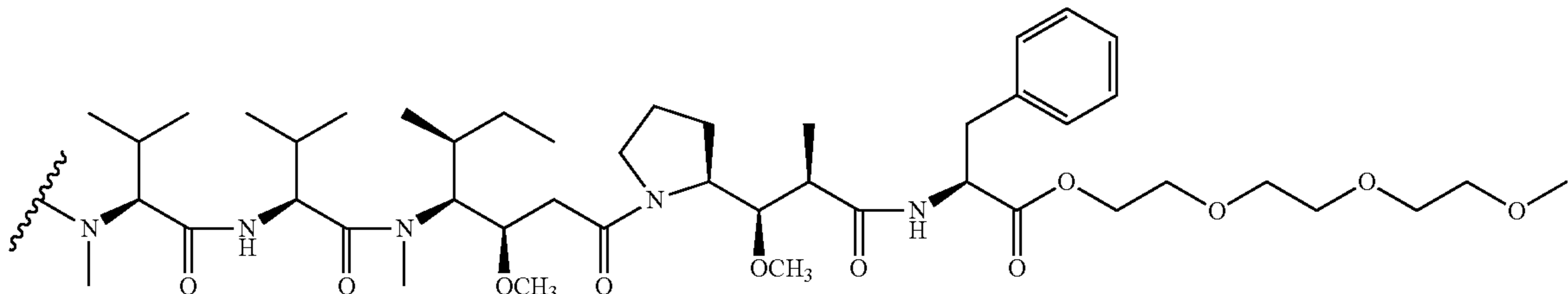
MMAF
