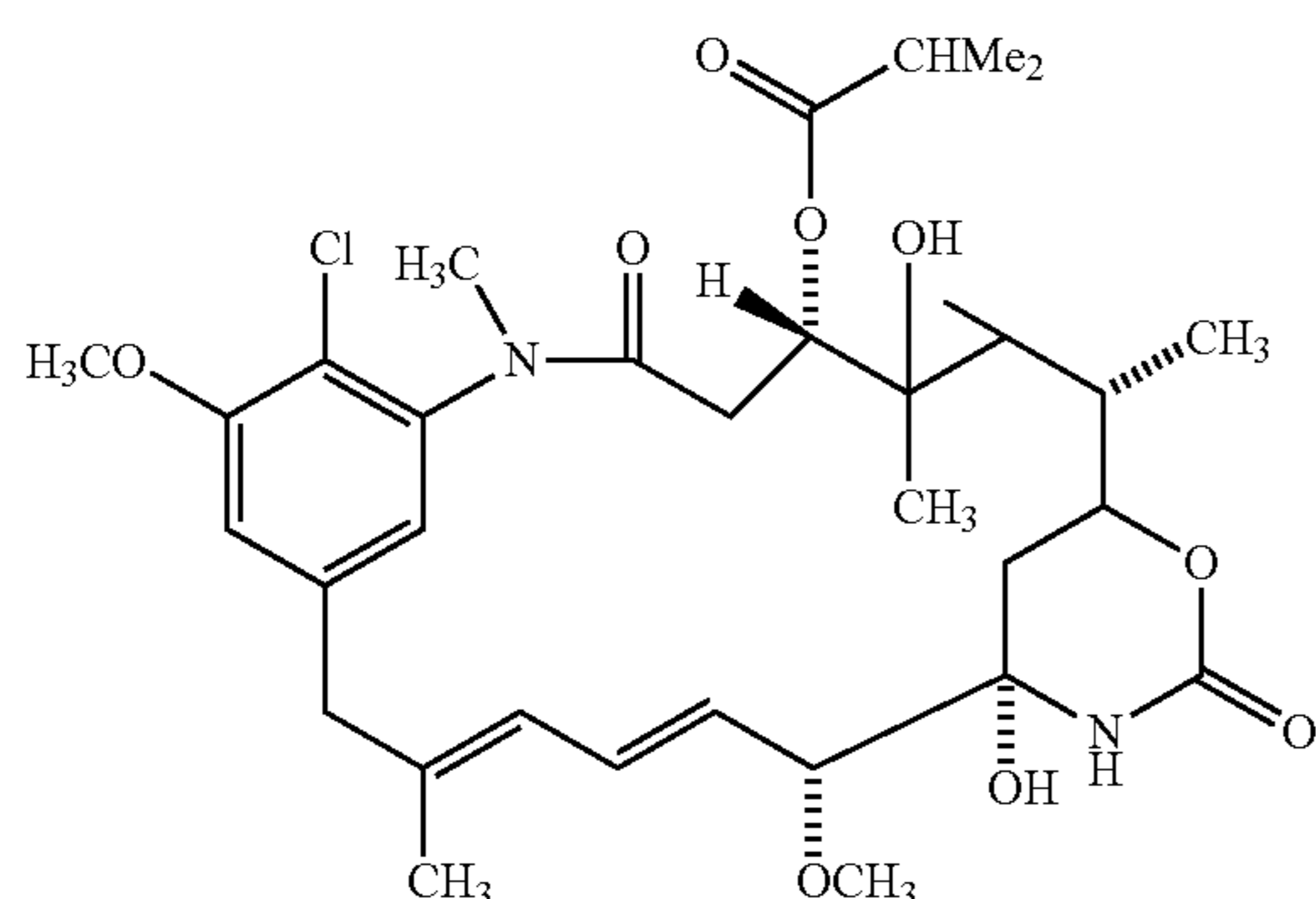
Ansamitocin P-3
