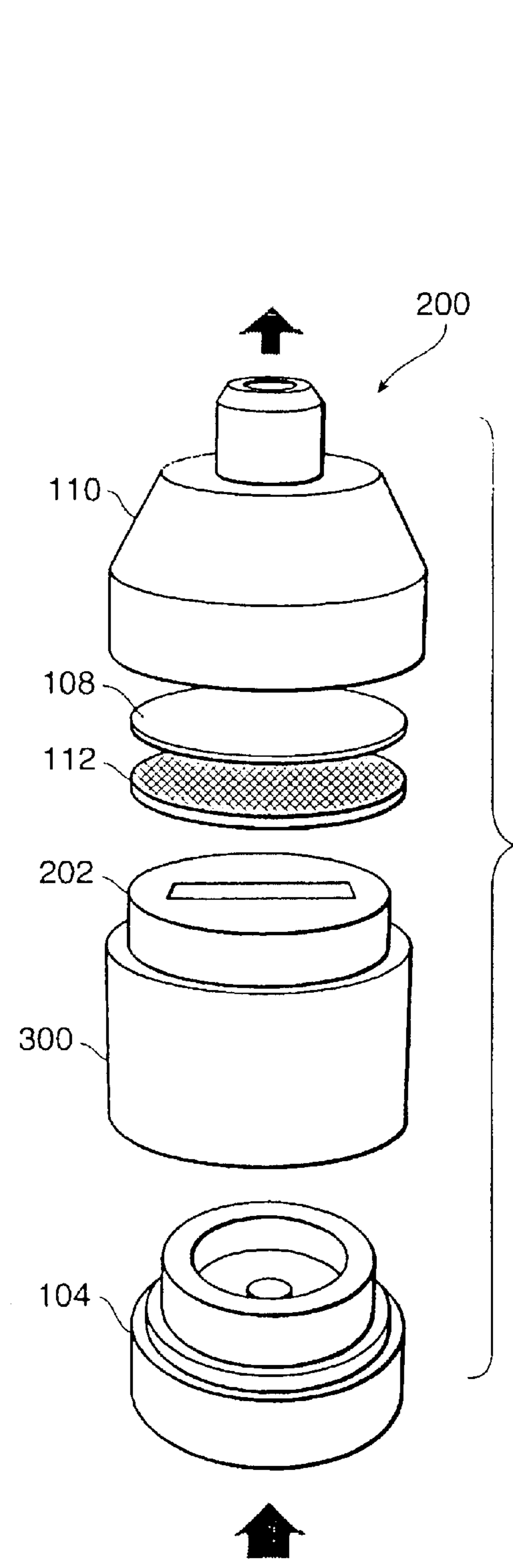
FIG. 4
