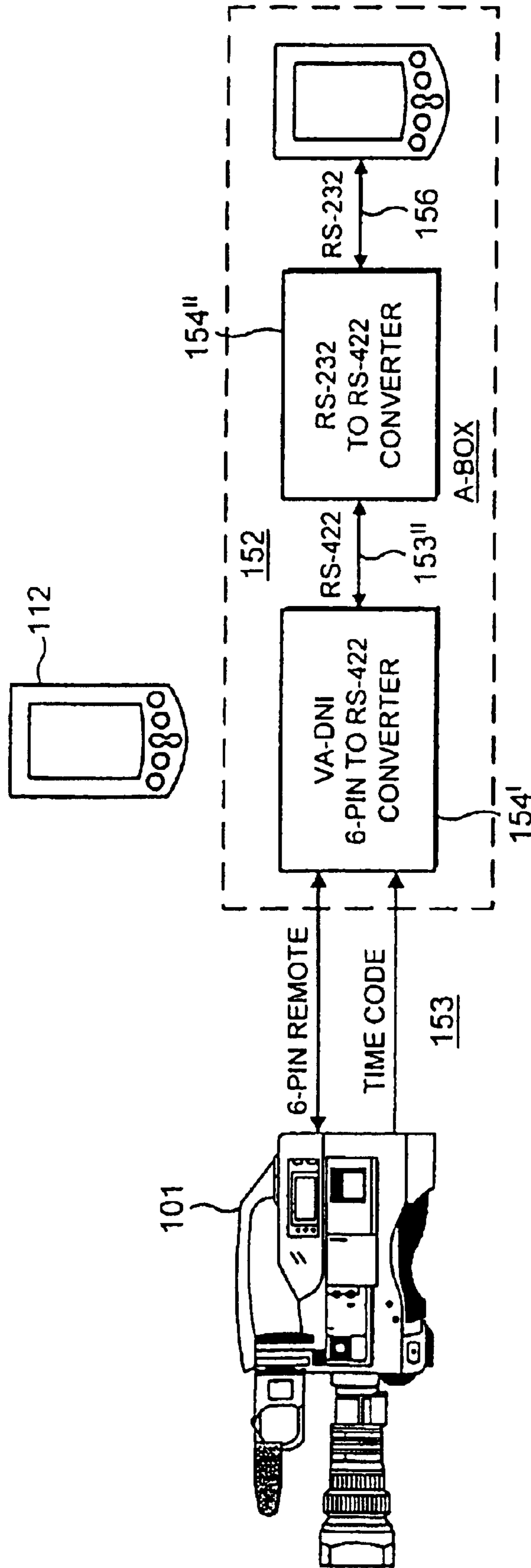
FIG. 6
