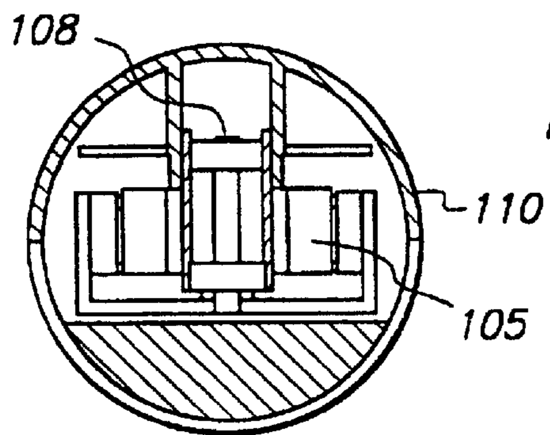
FIG. 1A (SECTION A-A)
