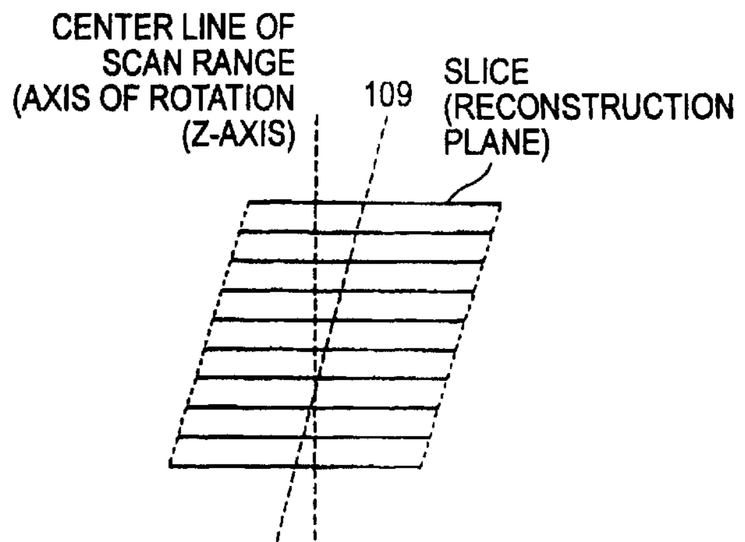
FIG. 8B
