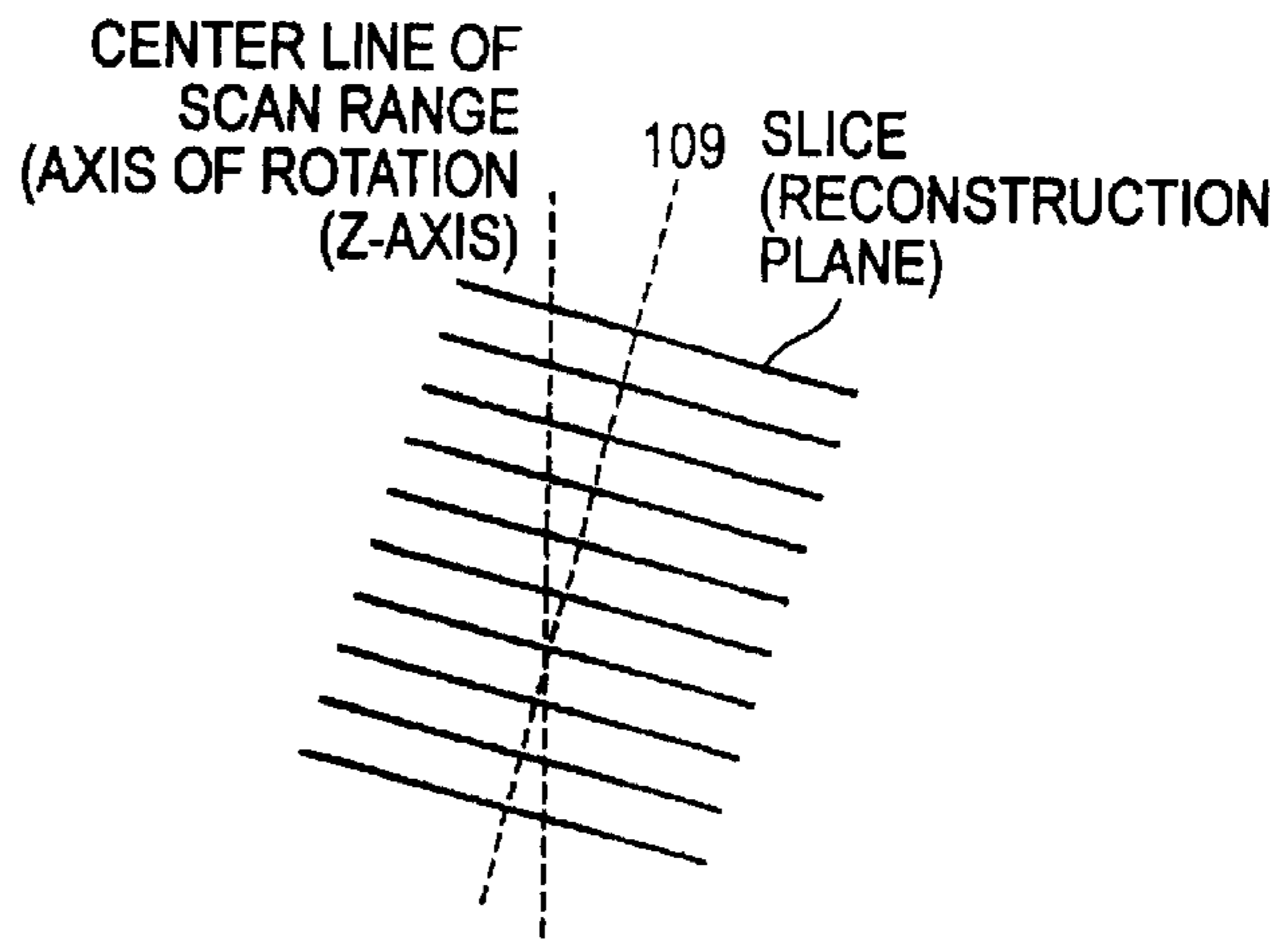
FIG. 9B
