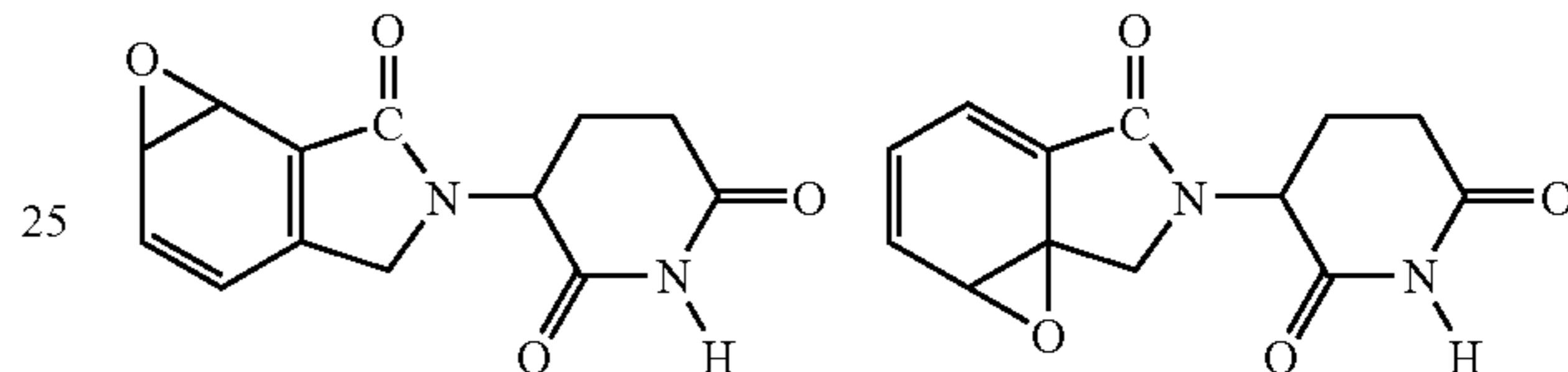
Epoxides of EM 12
