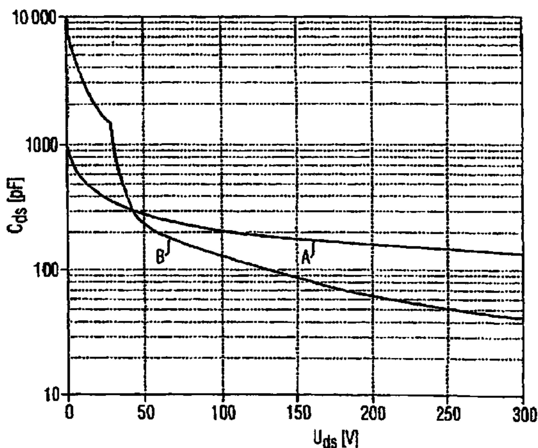
A: Standard-MOSFET B: Inventive MOSFET
