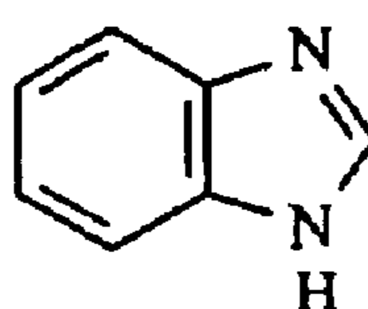
benzimidazole
