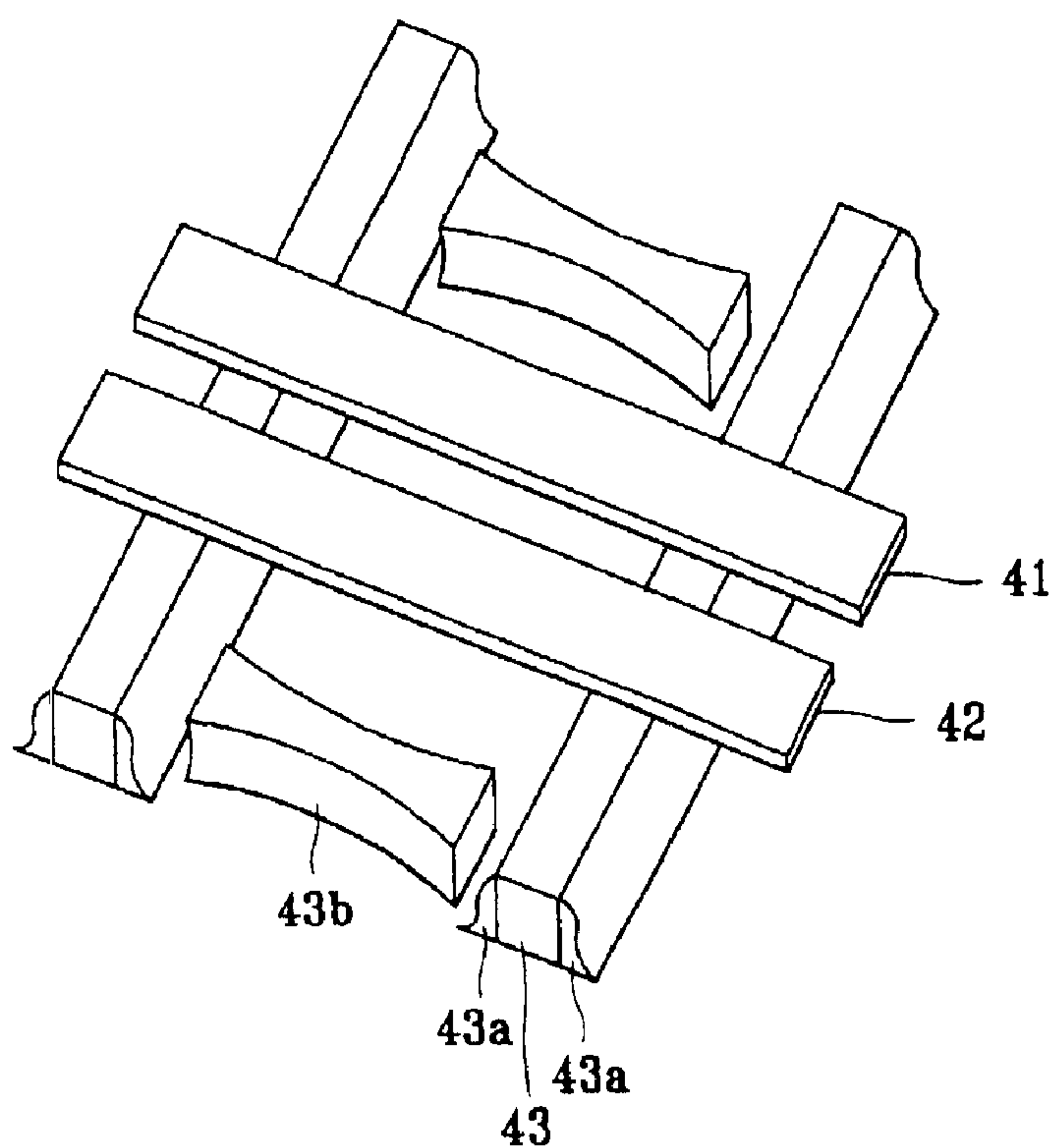
FIG.4b
