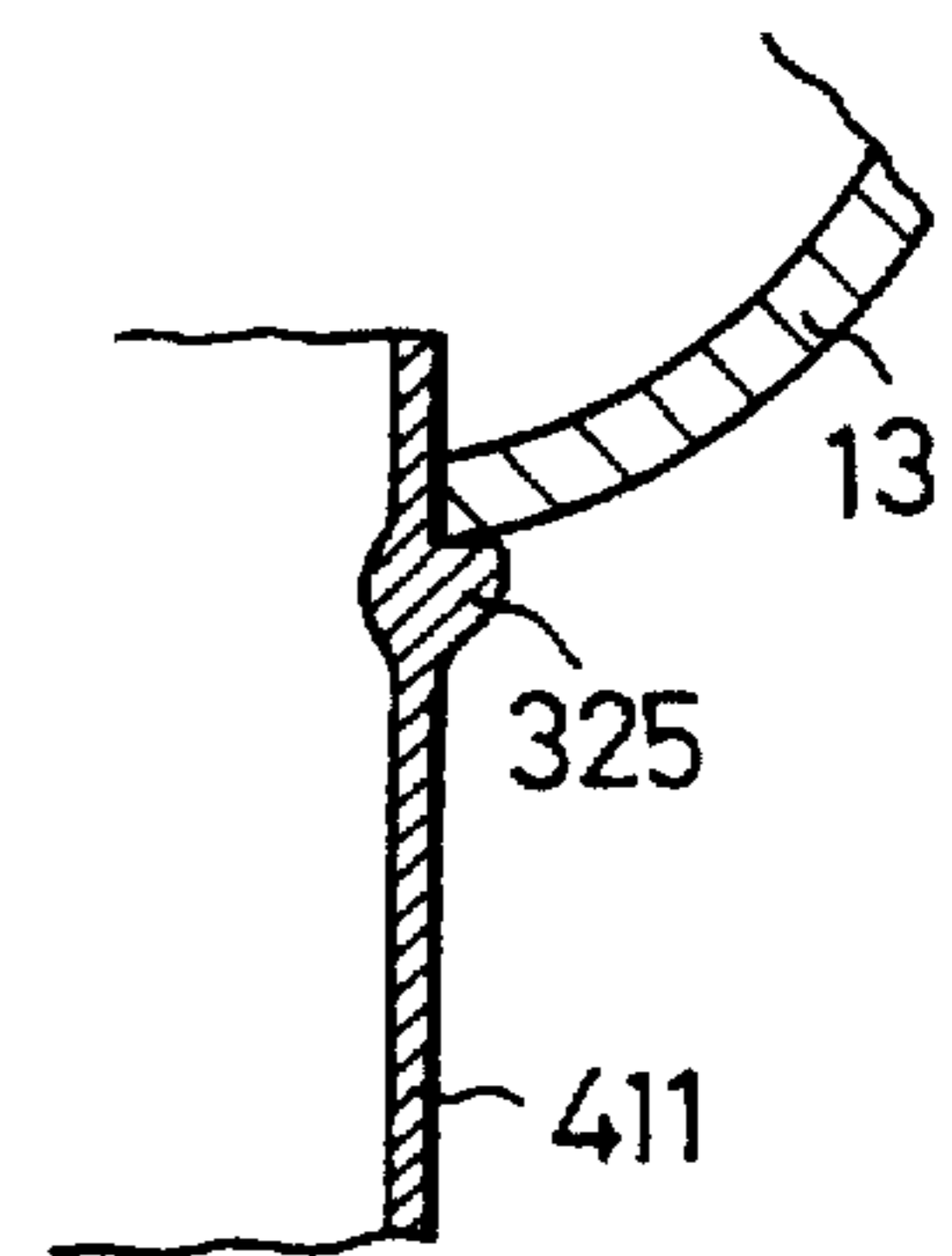
FIG. 13C
