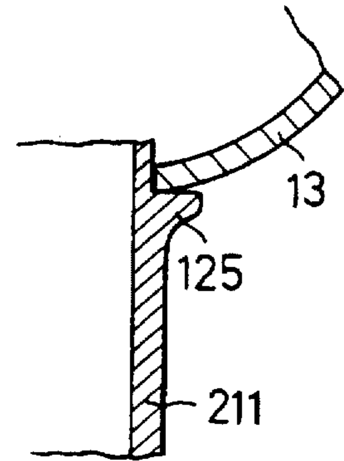
FIG. 11C
