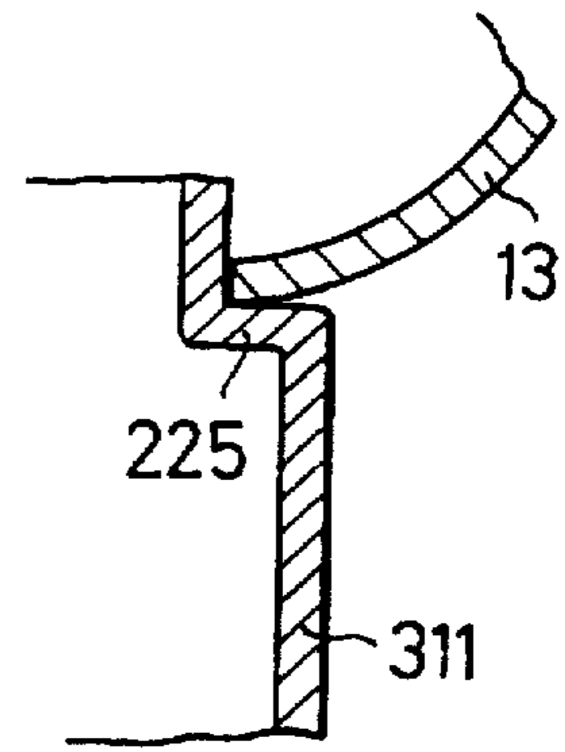
FIG. 12C
