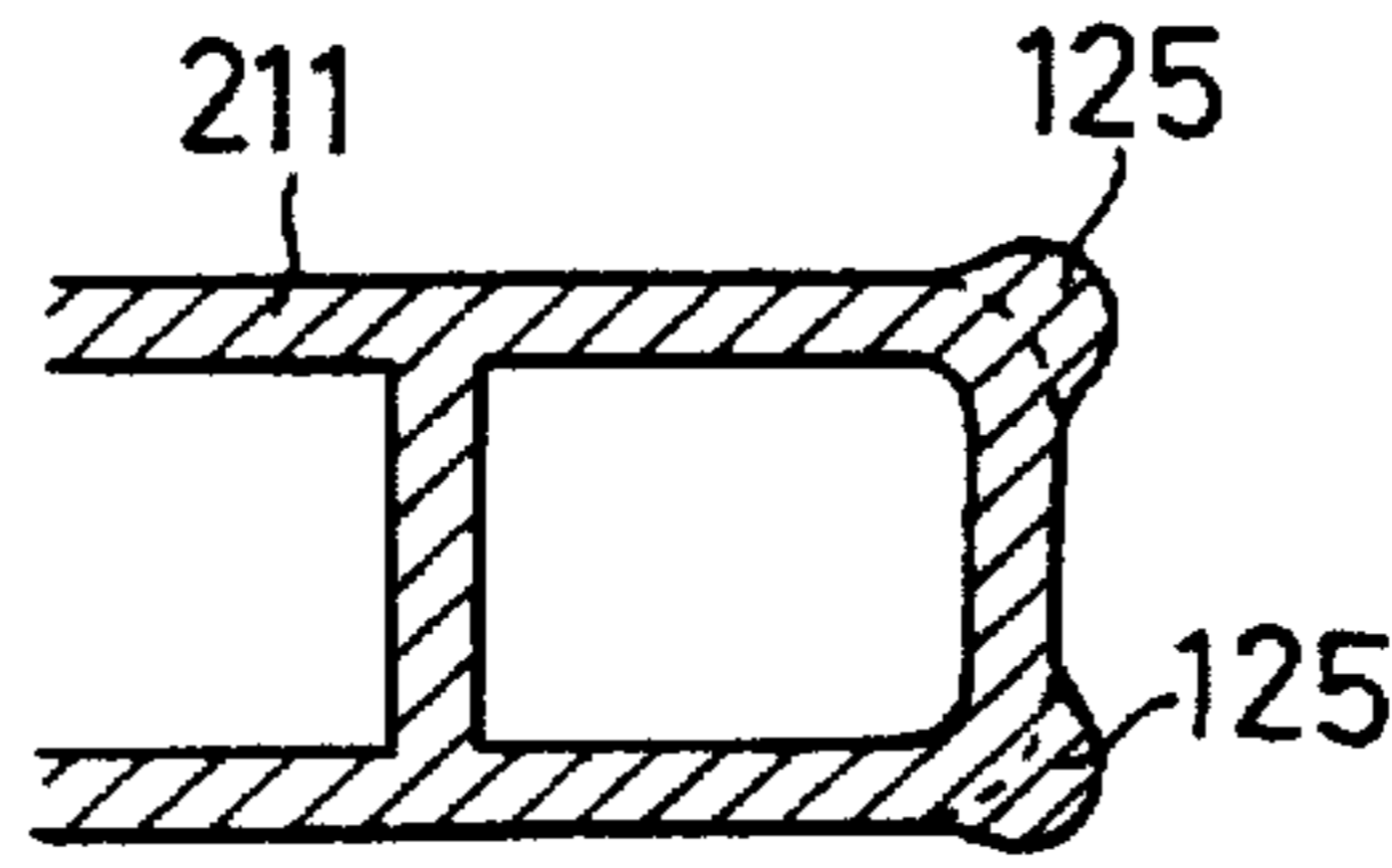
FIG. 11B
