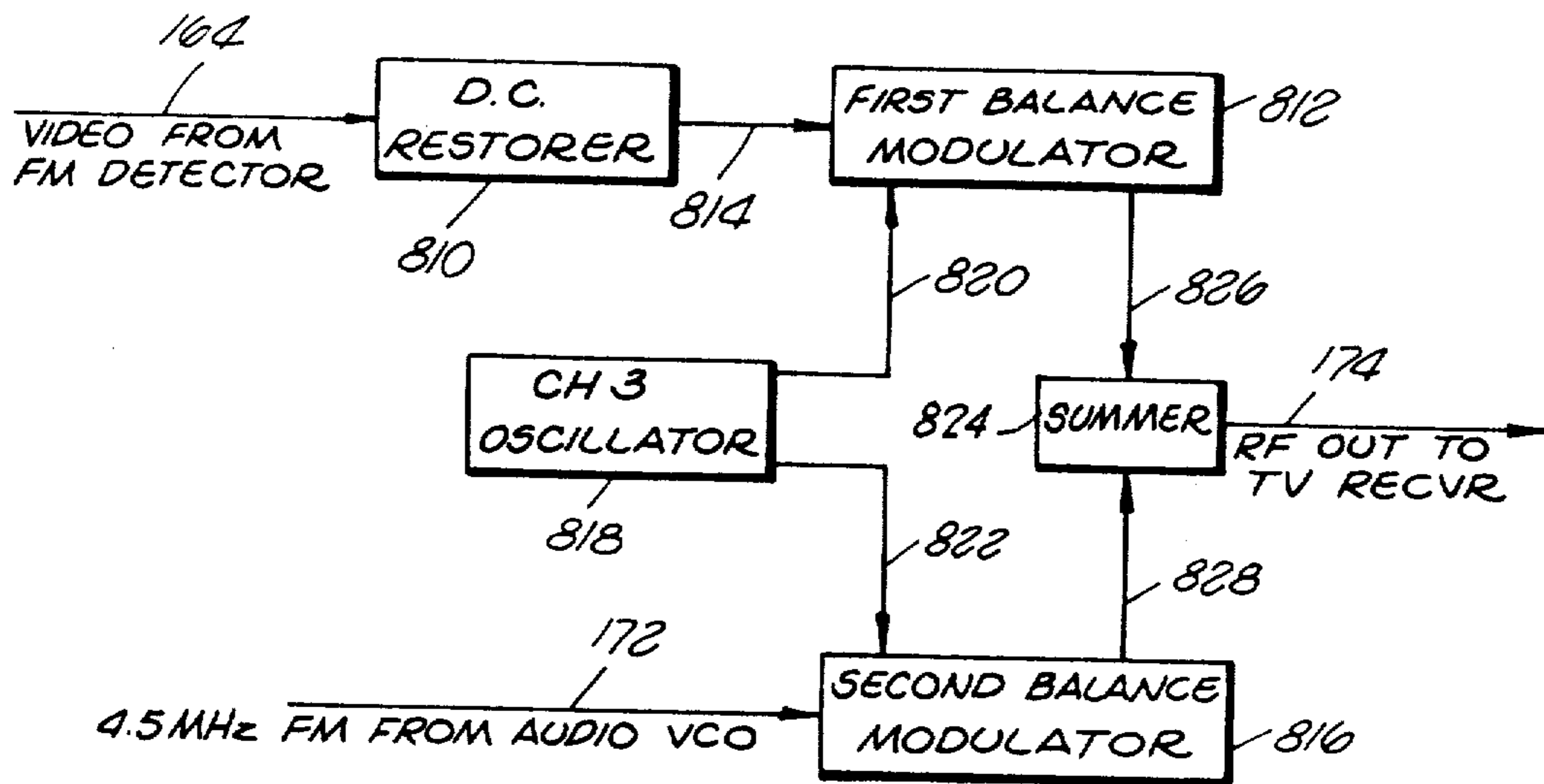
FIG. 24 RF MODULATOR
