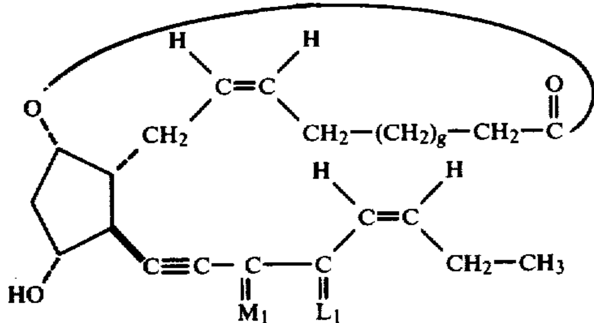
13,14-didehydro-PGF 3α -type, 1,9-lactones
