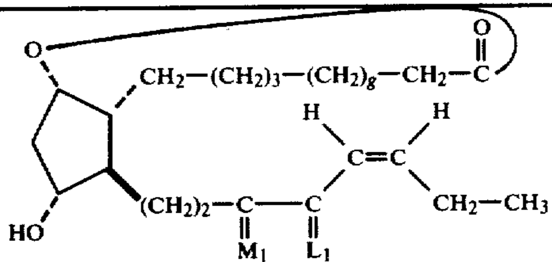
5,6,13,14-tetrahydro-PGF 3α -type, 1,9-lactones
