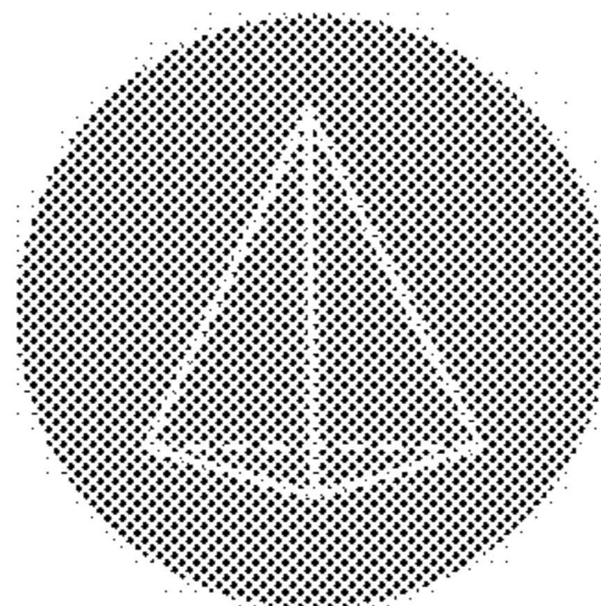
PYRAMID
