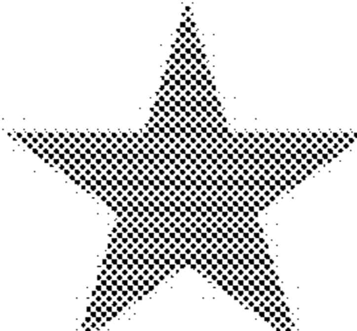
STAR
