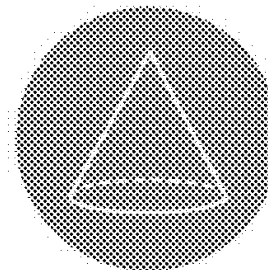
CONE
