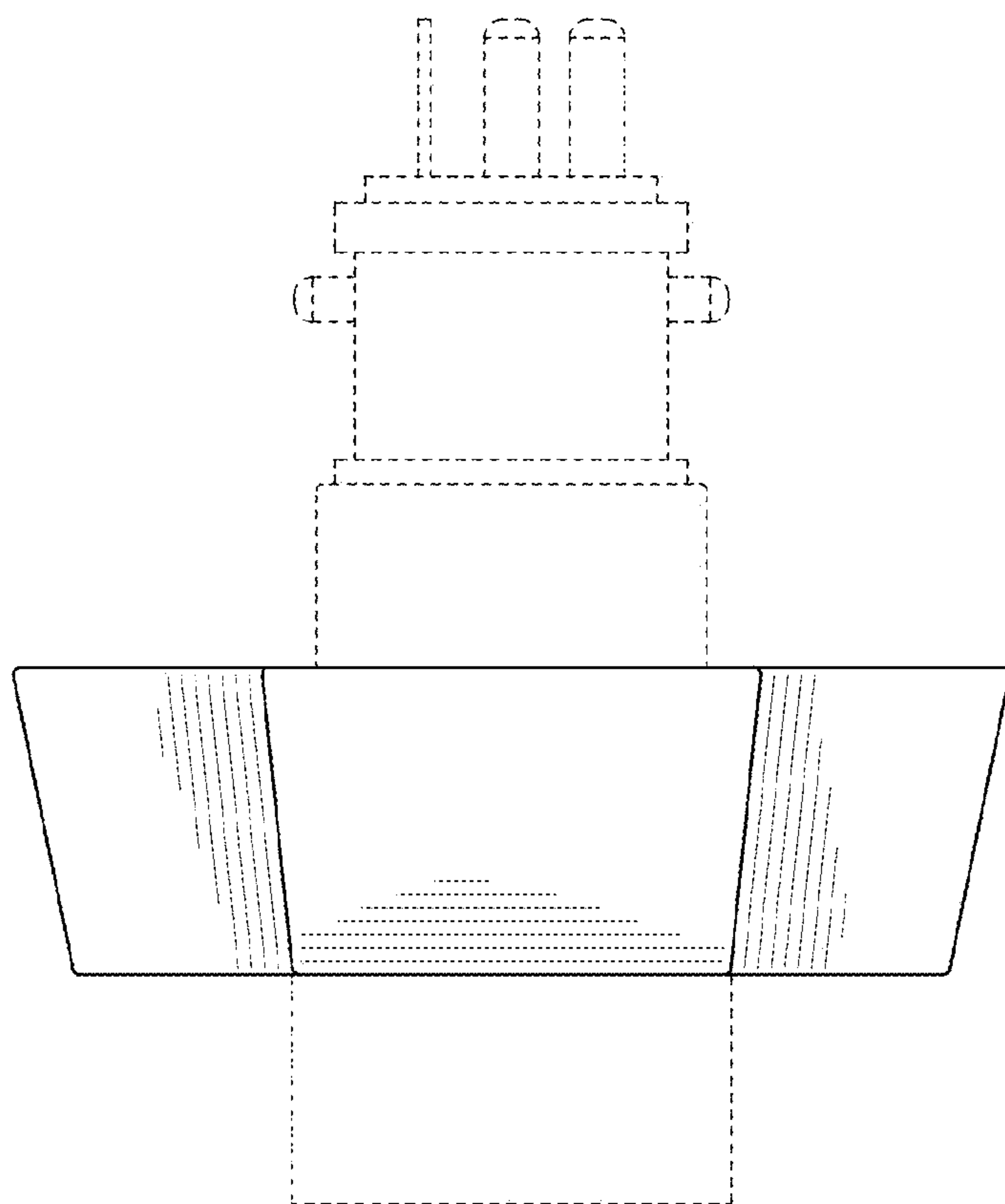
FIG. 3
