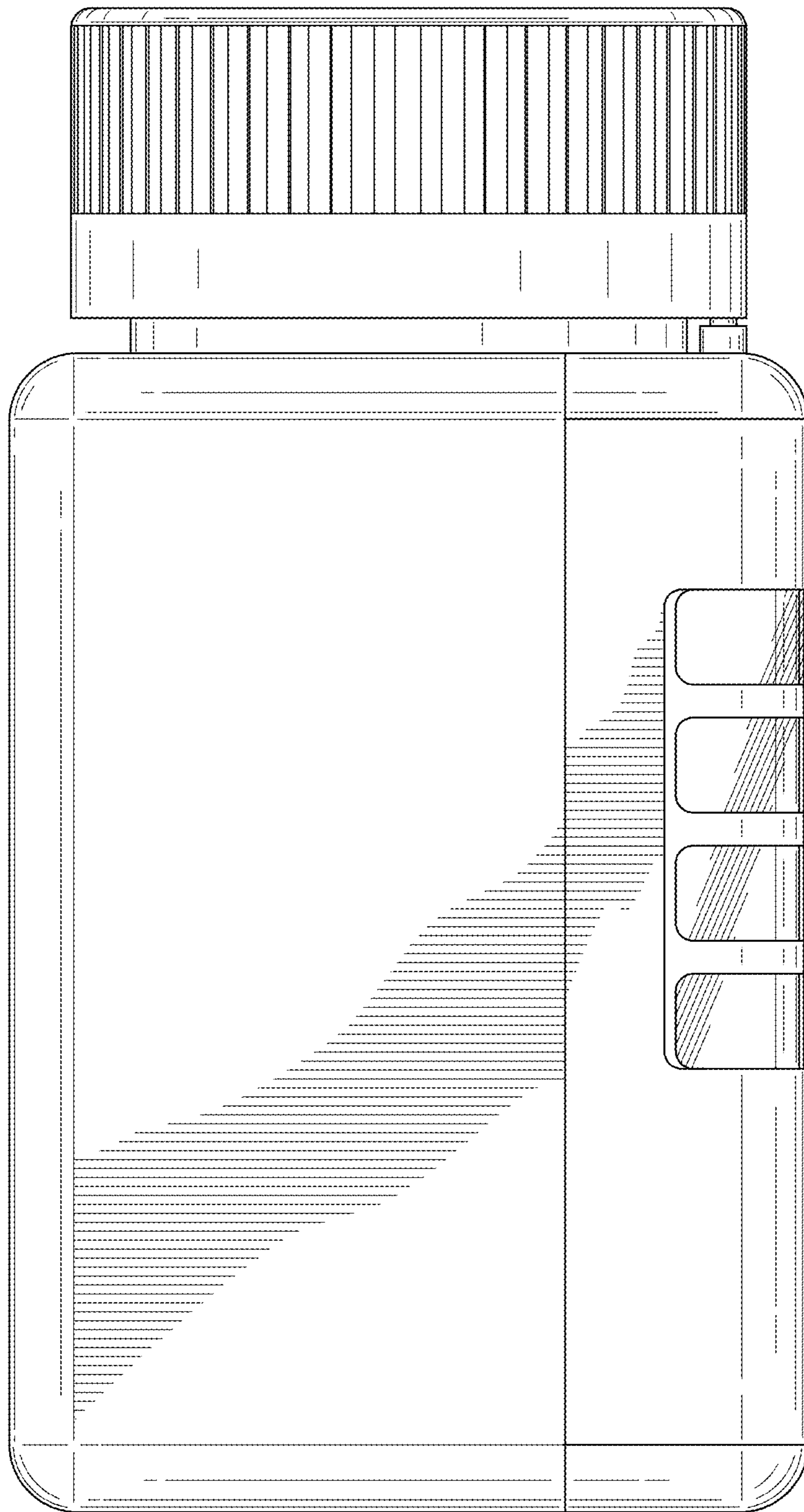
FIG. 4
