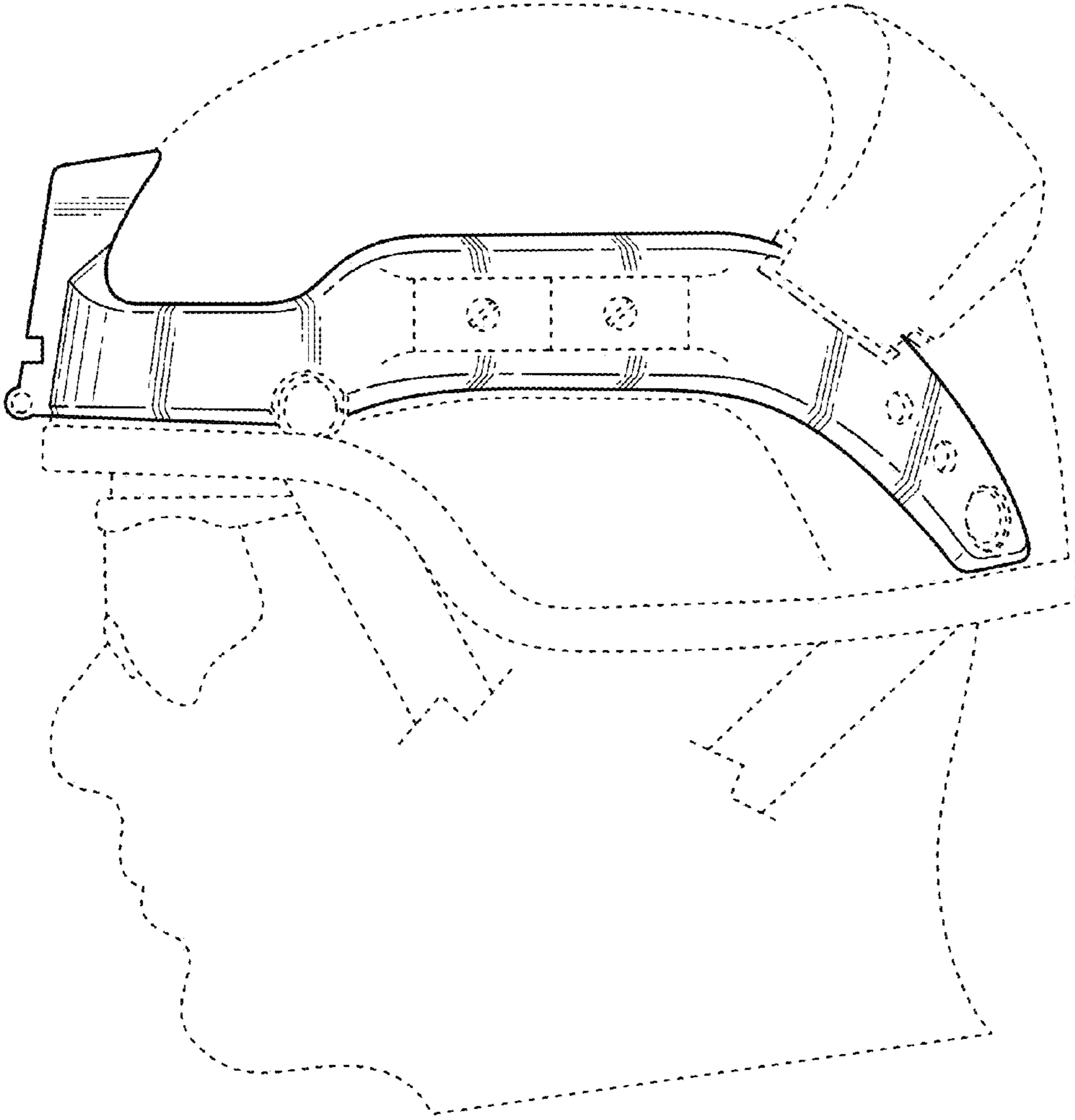
FIG. 2
