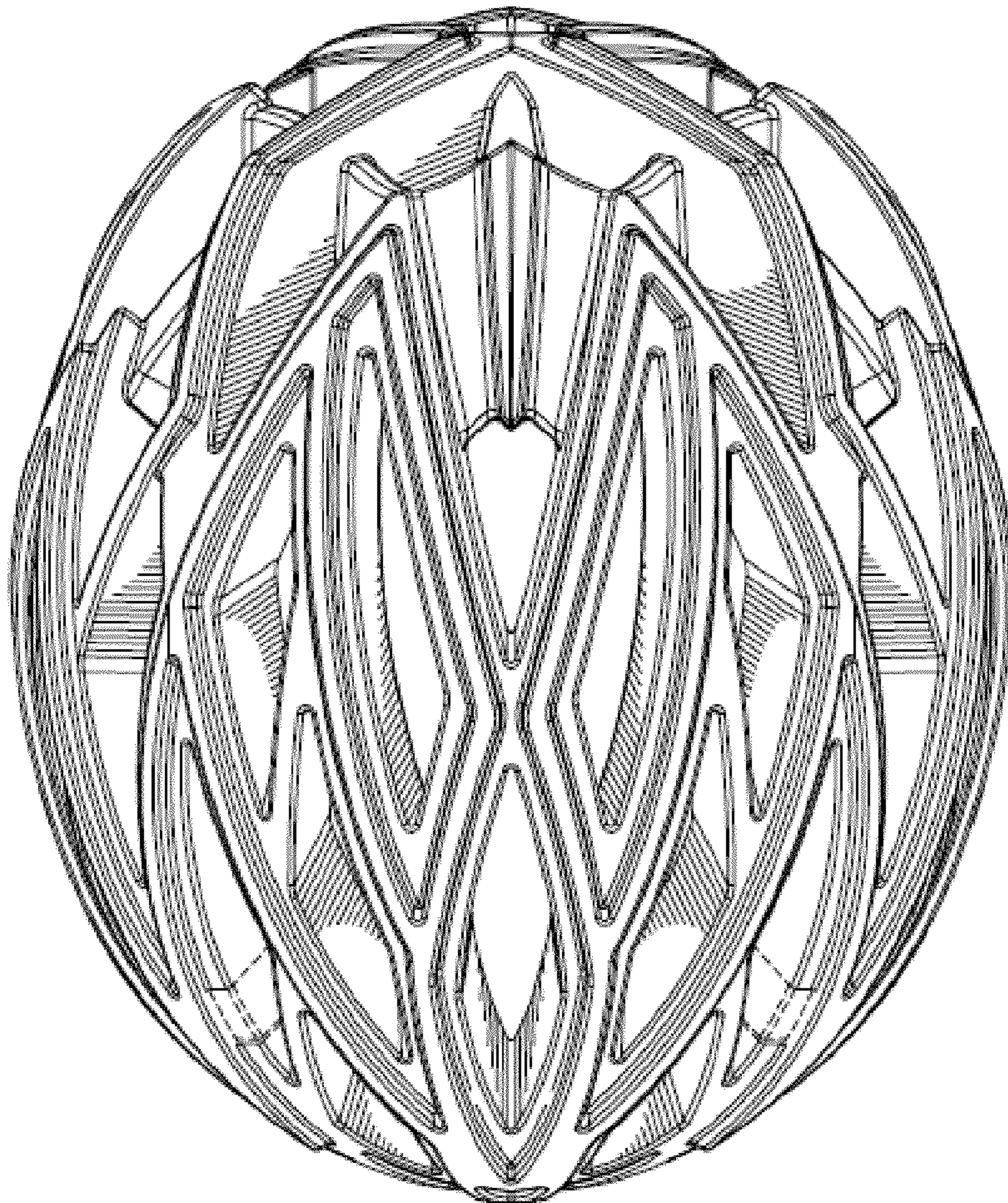
FIG. 5
