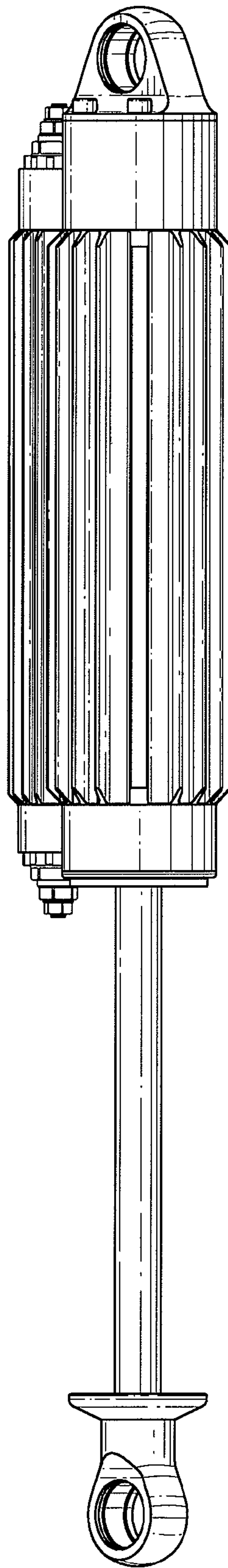
FIG. 1
