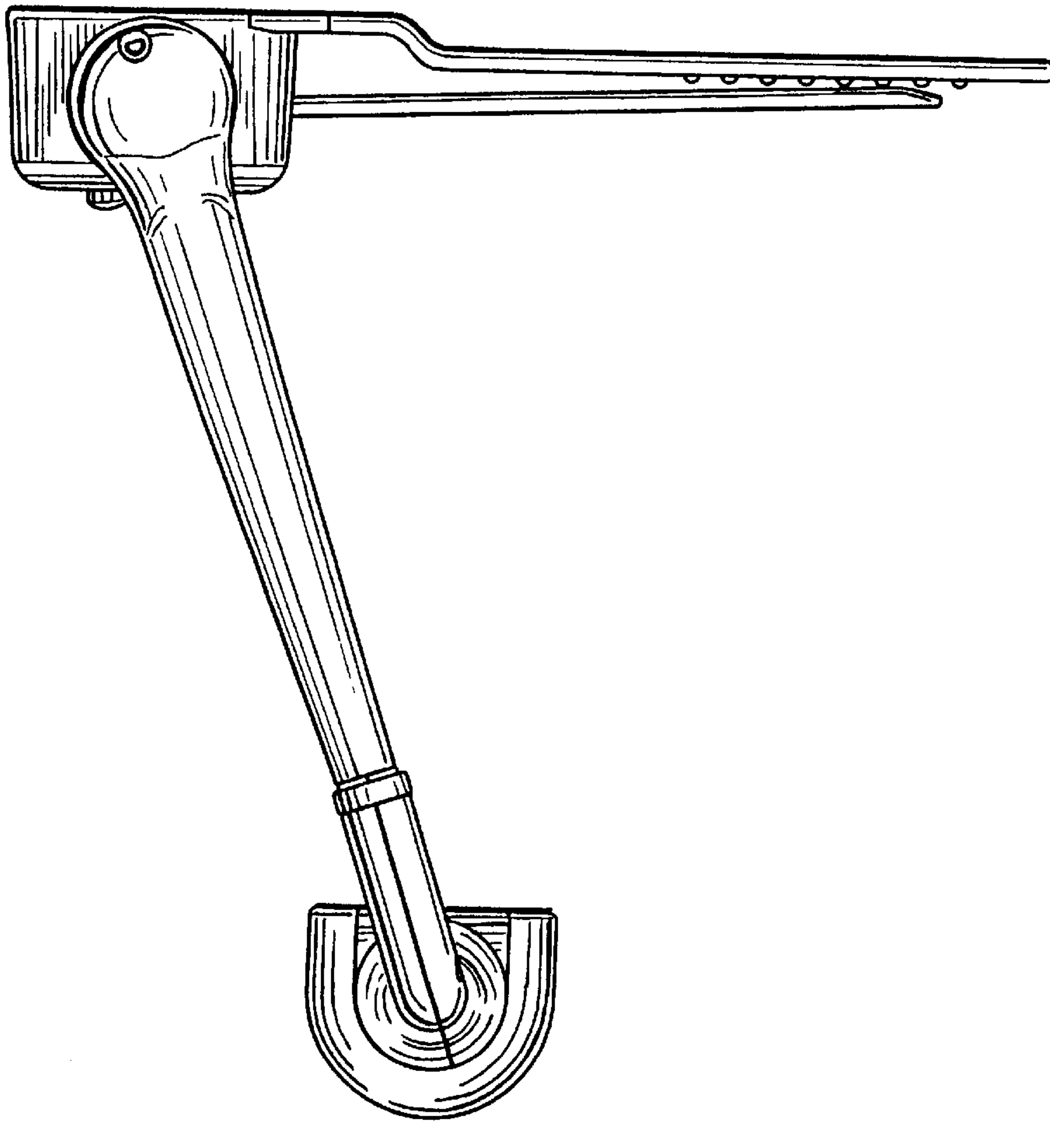
FIG. 4
