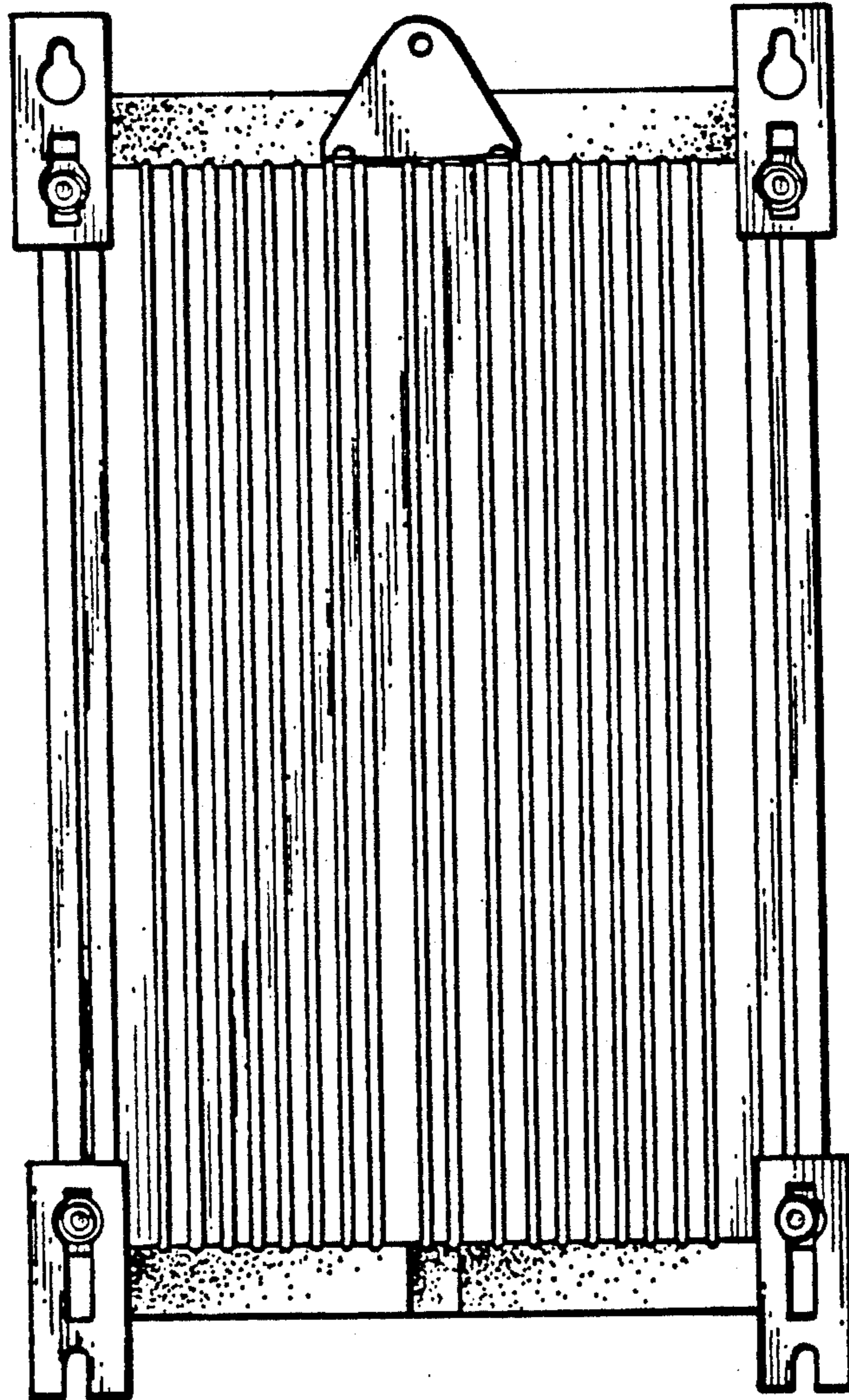
FIG. 5
