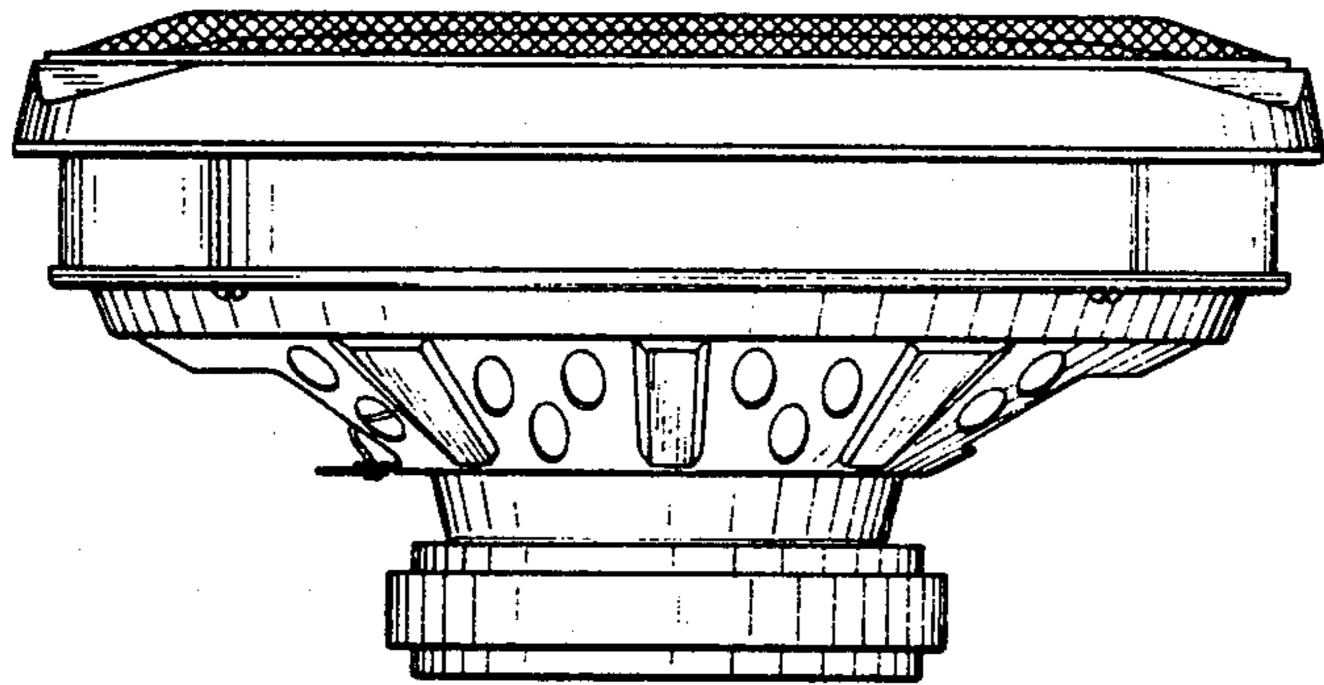
FIG. 6
