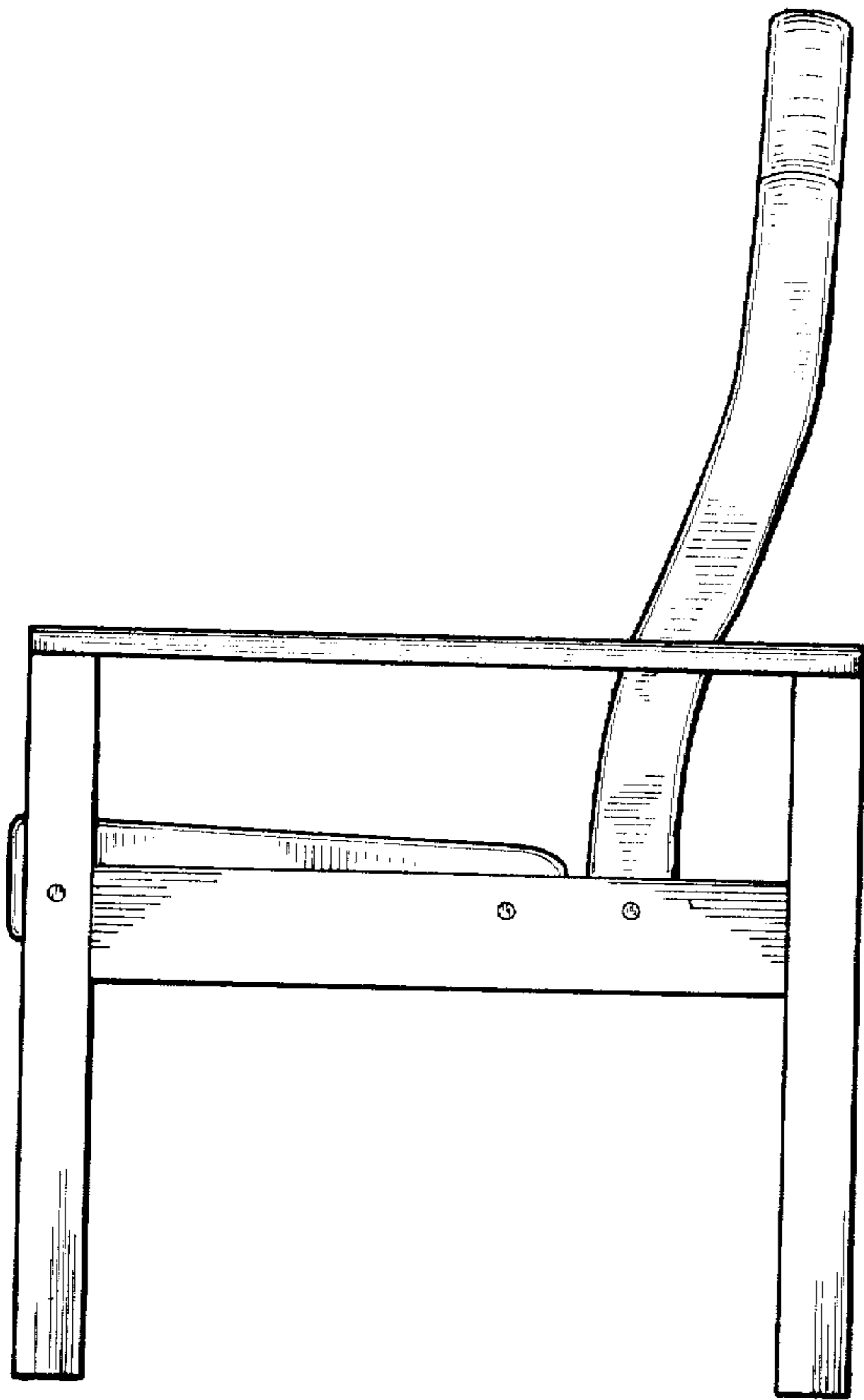
FIG. 3
