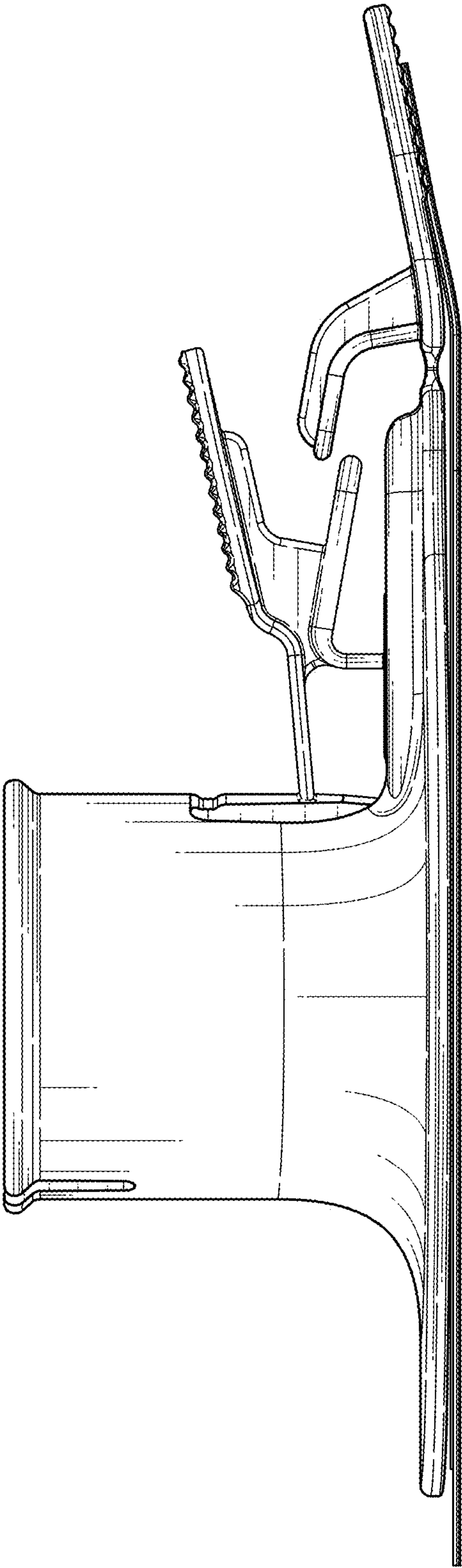
FIG. 5
