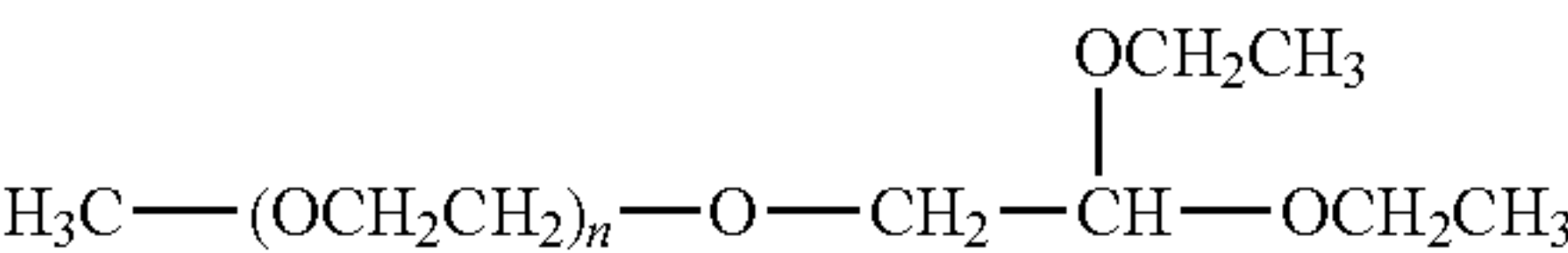
mPEG Acetal
