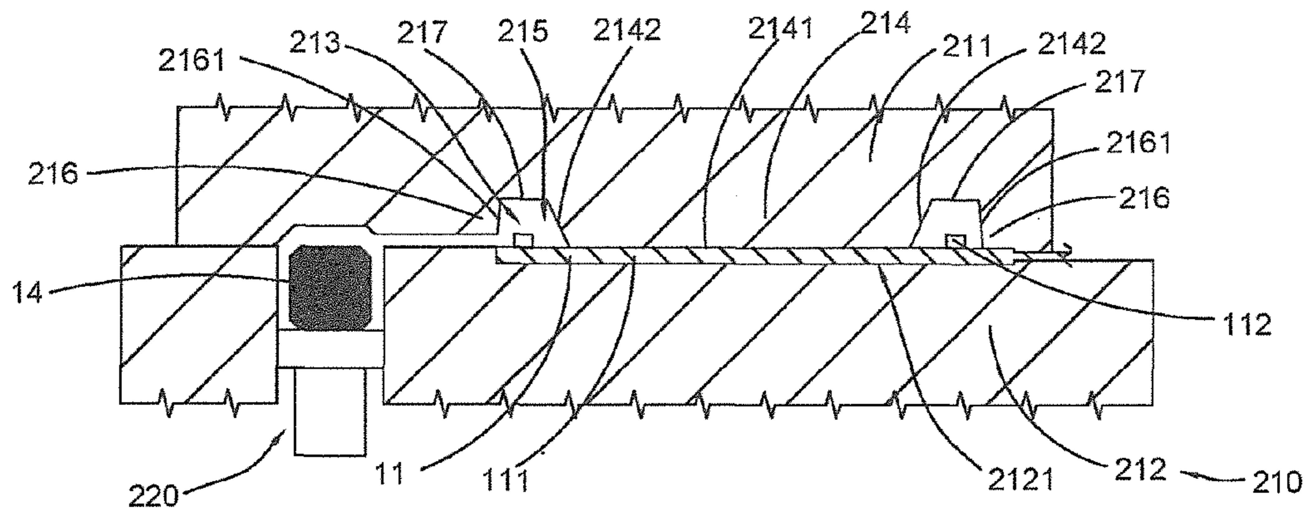
A-A FIG. 8A
