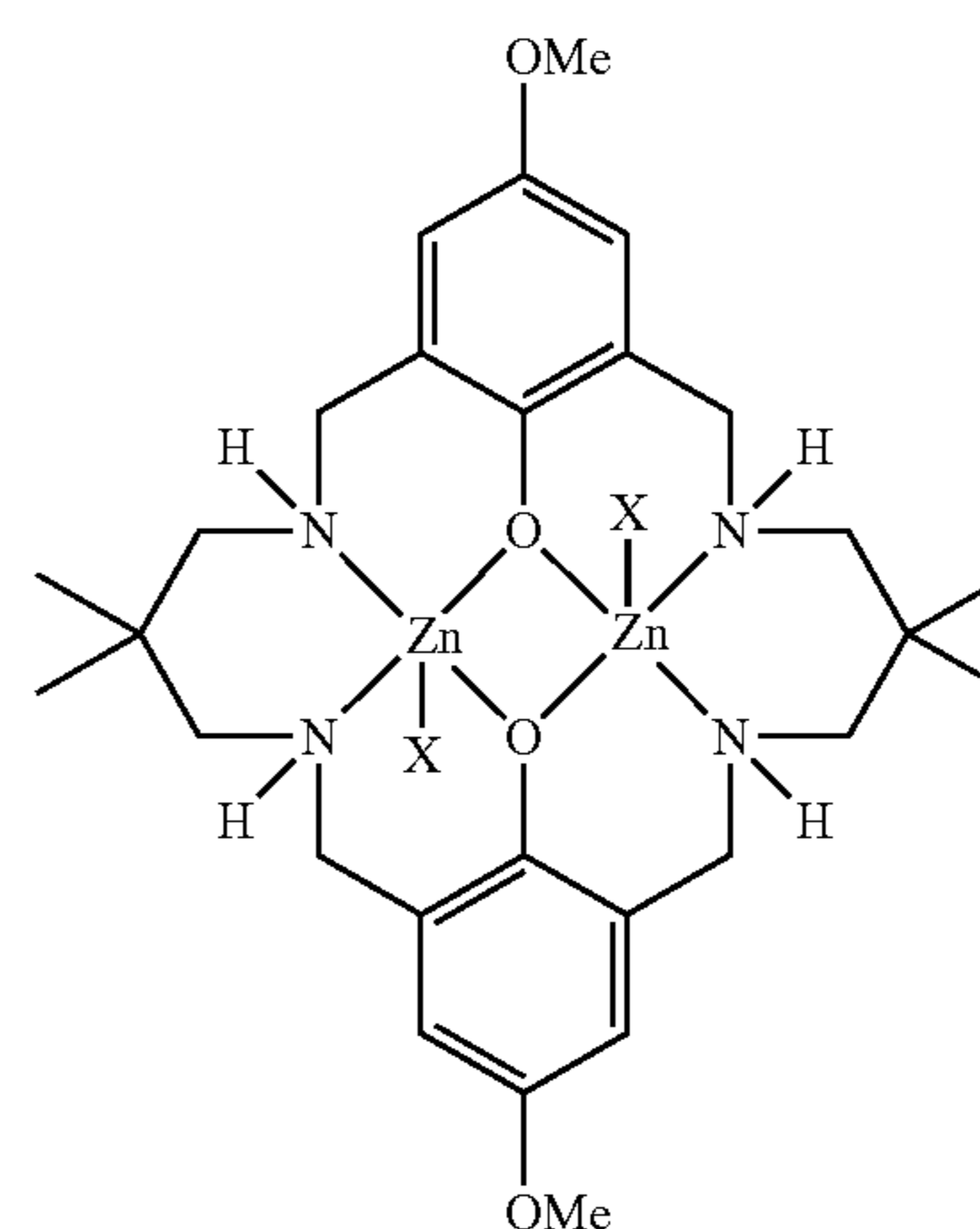
L 3 Zn 2 (OAc) 2
