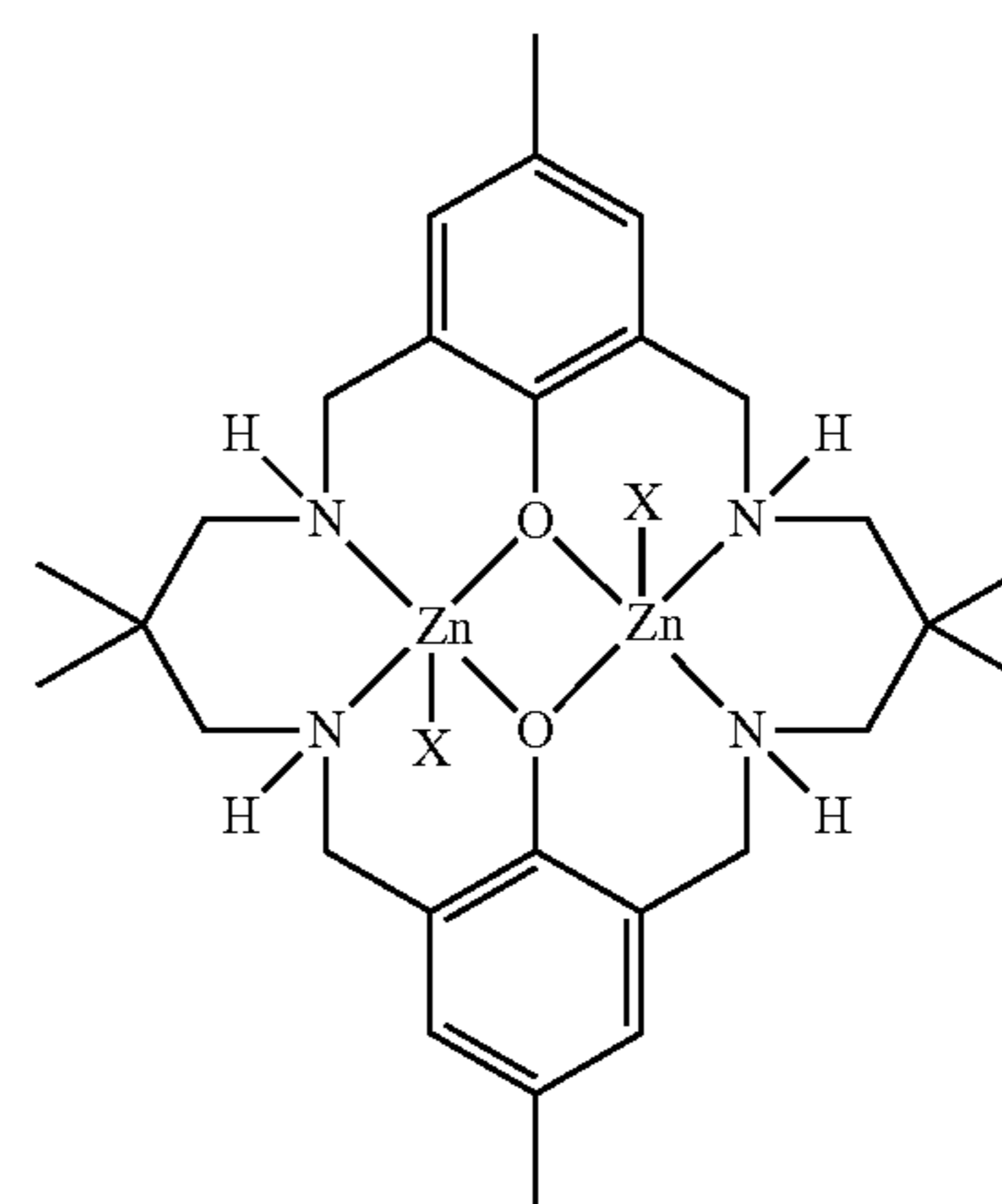
L 2 Zn 2 (OAc) 2
