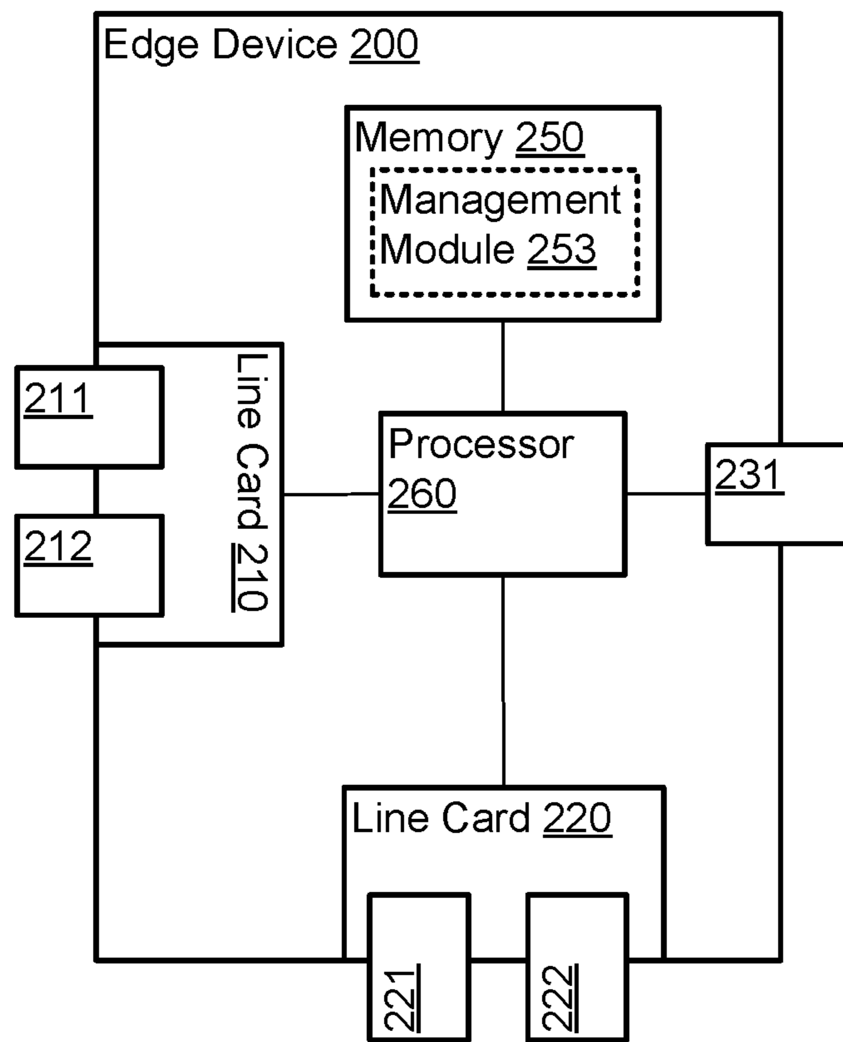
FIG. 2
