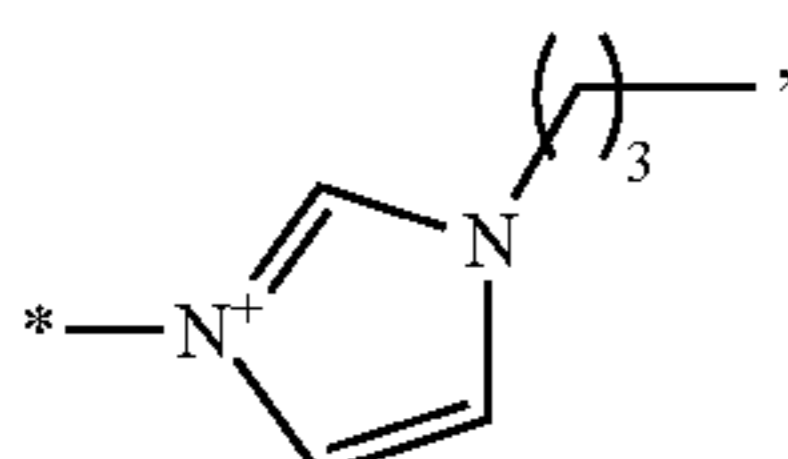
(butyl imidazolium)
