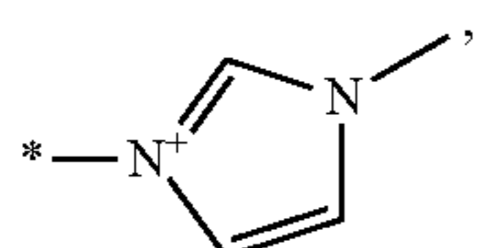
(methyl imidazolium)
