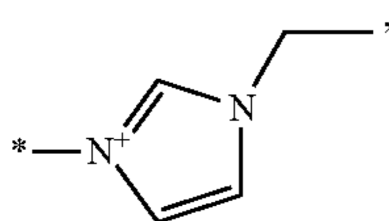
(ethyl imidazolium)
