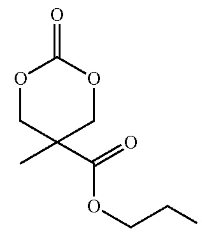
(MTC-EtI)
