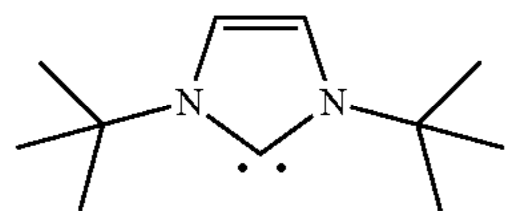
1,3-Di-t-butylimidazol-2-ylidene (Im-6)
