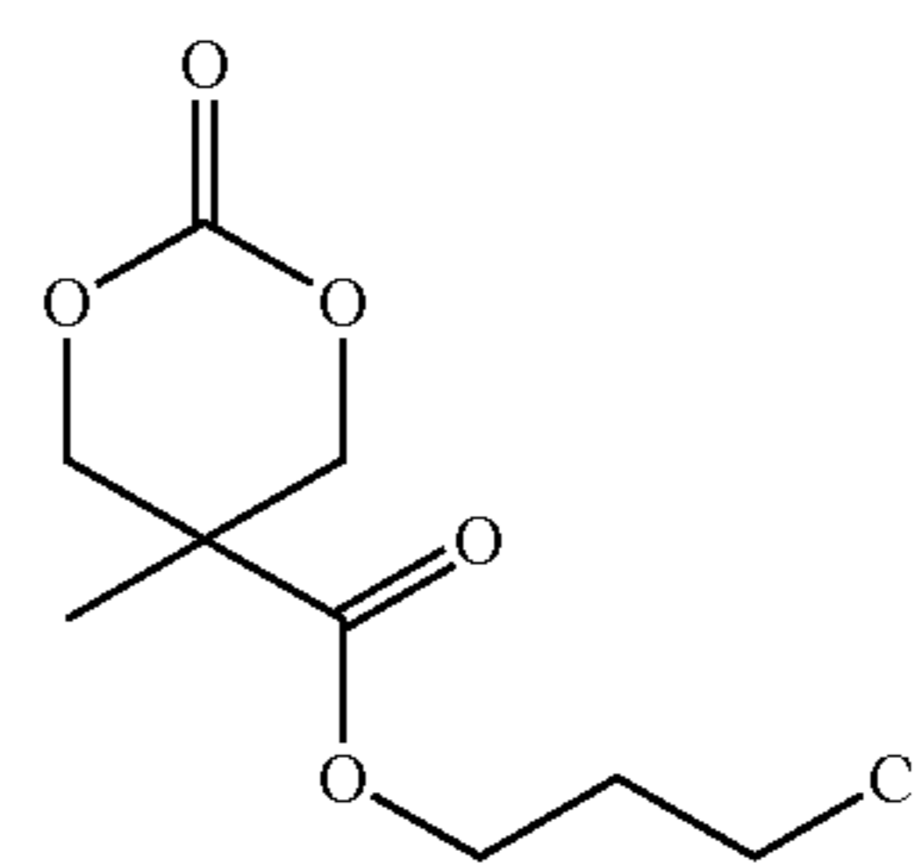
(MTC-PrCl)
