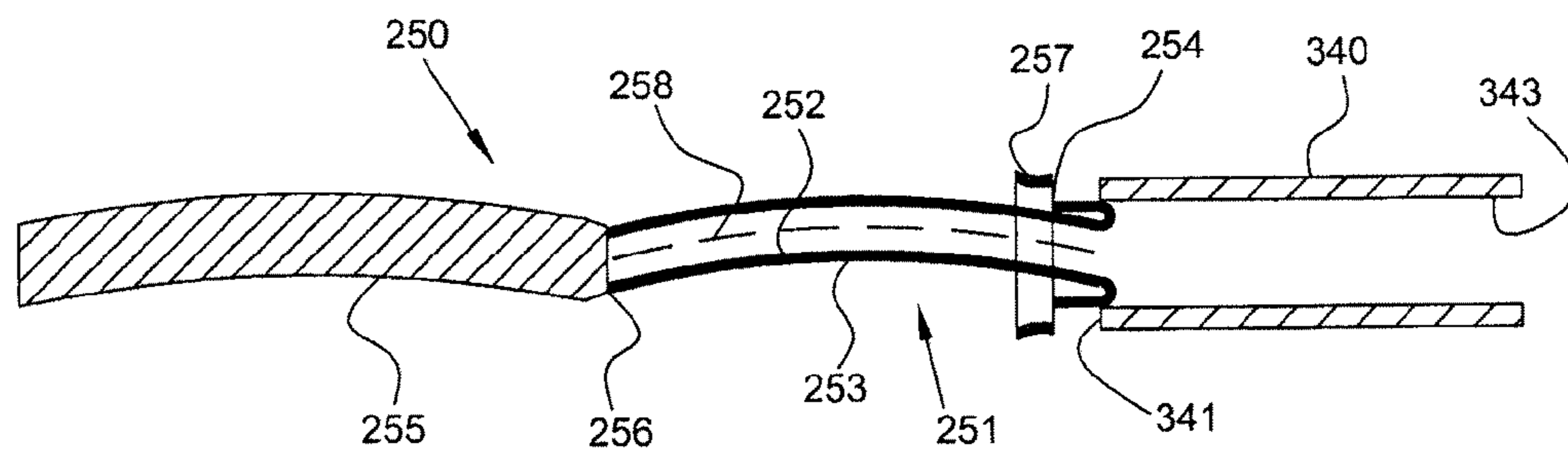
FIG 3A
