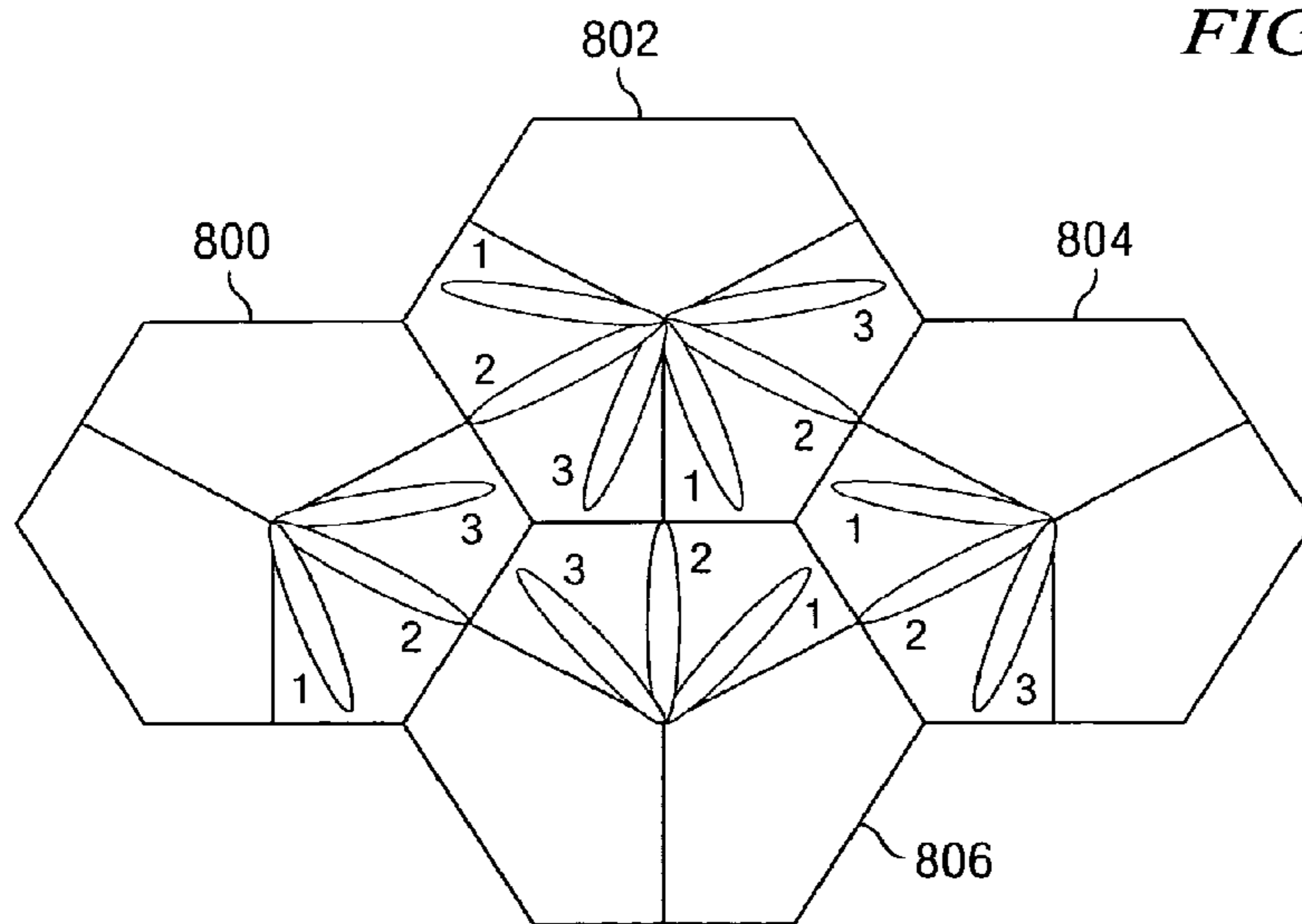
FIG. 8
