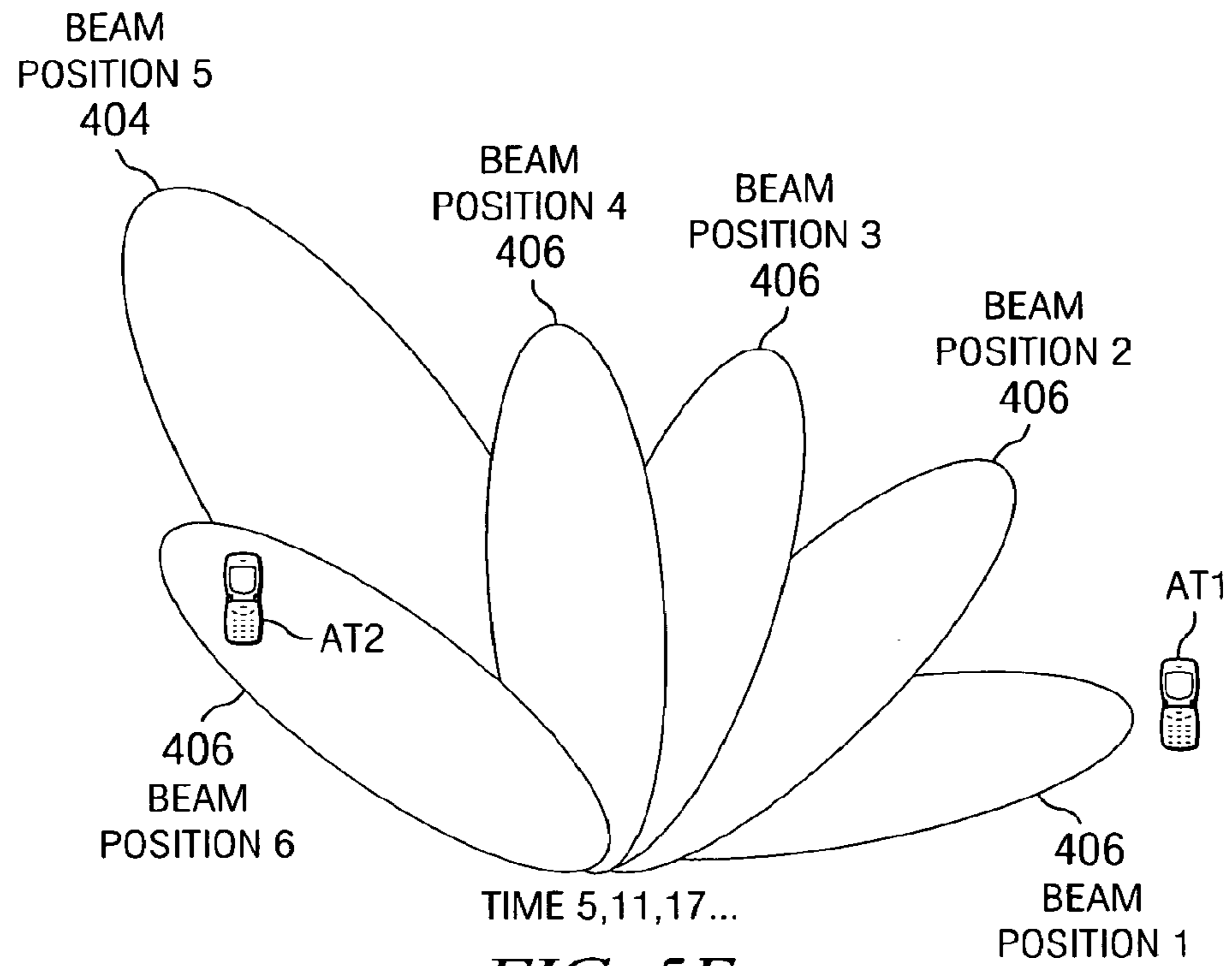
FIG. 5E
