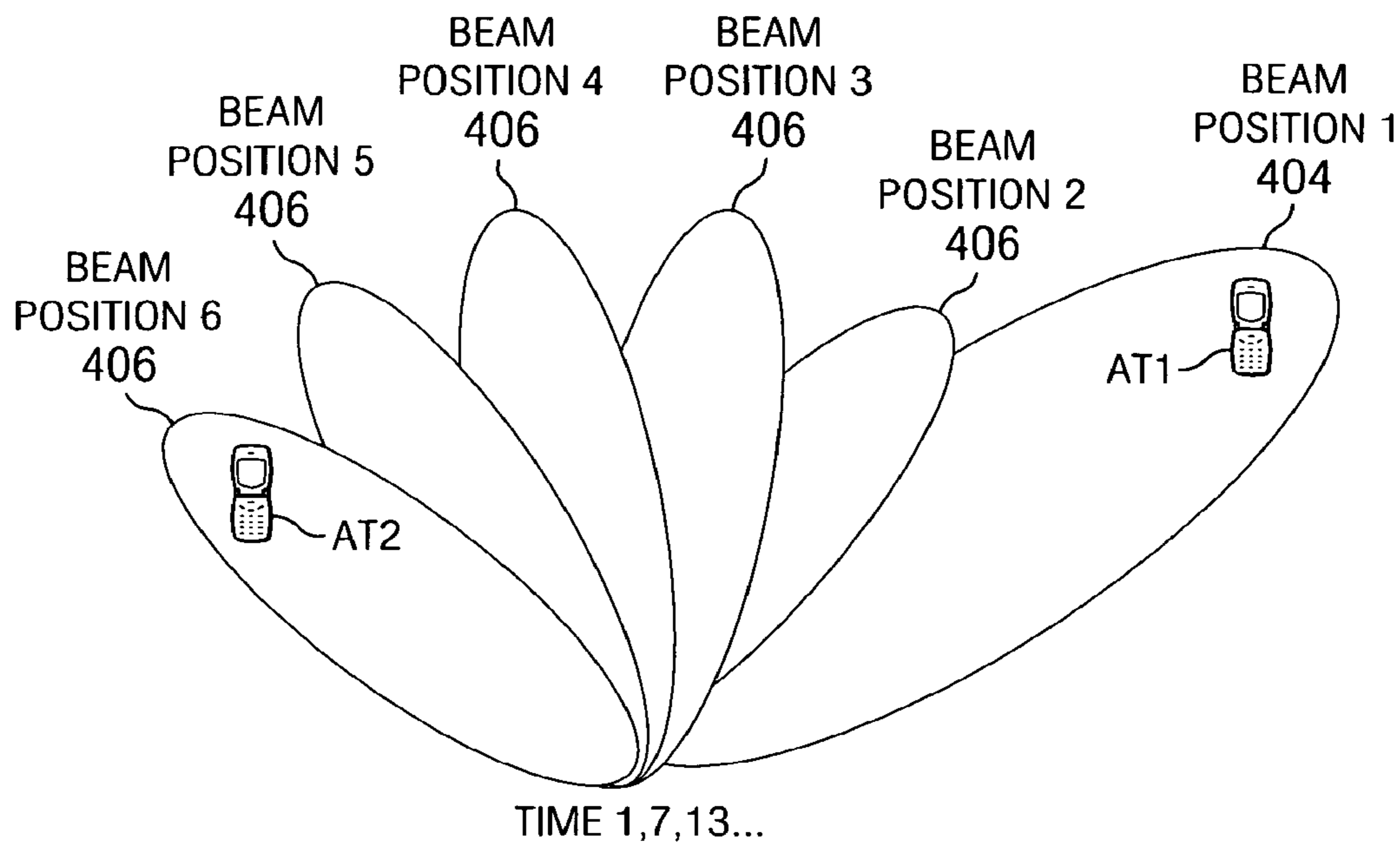
FIG. 5A
