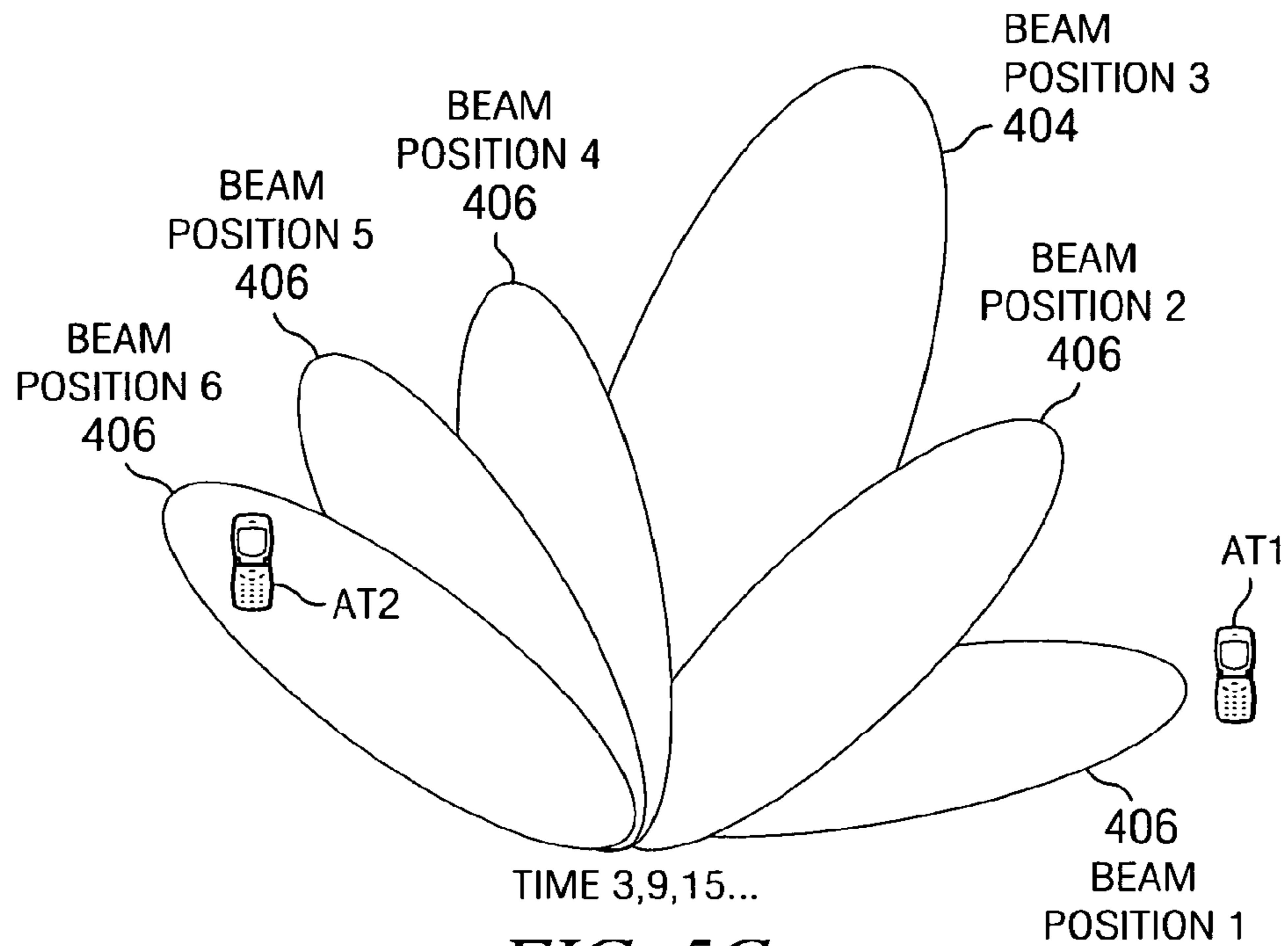
FIG. 5C
