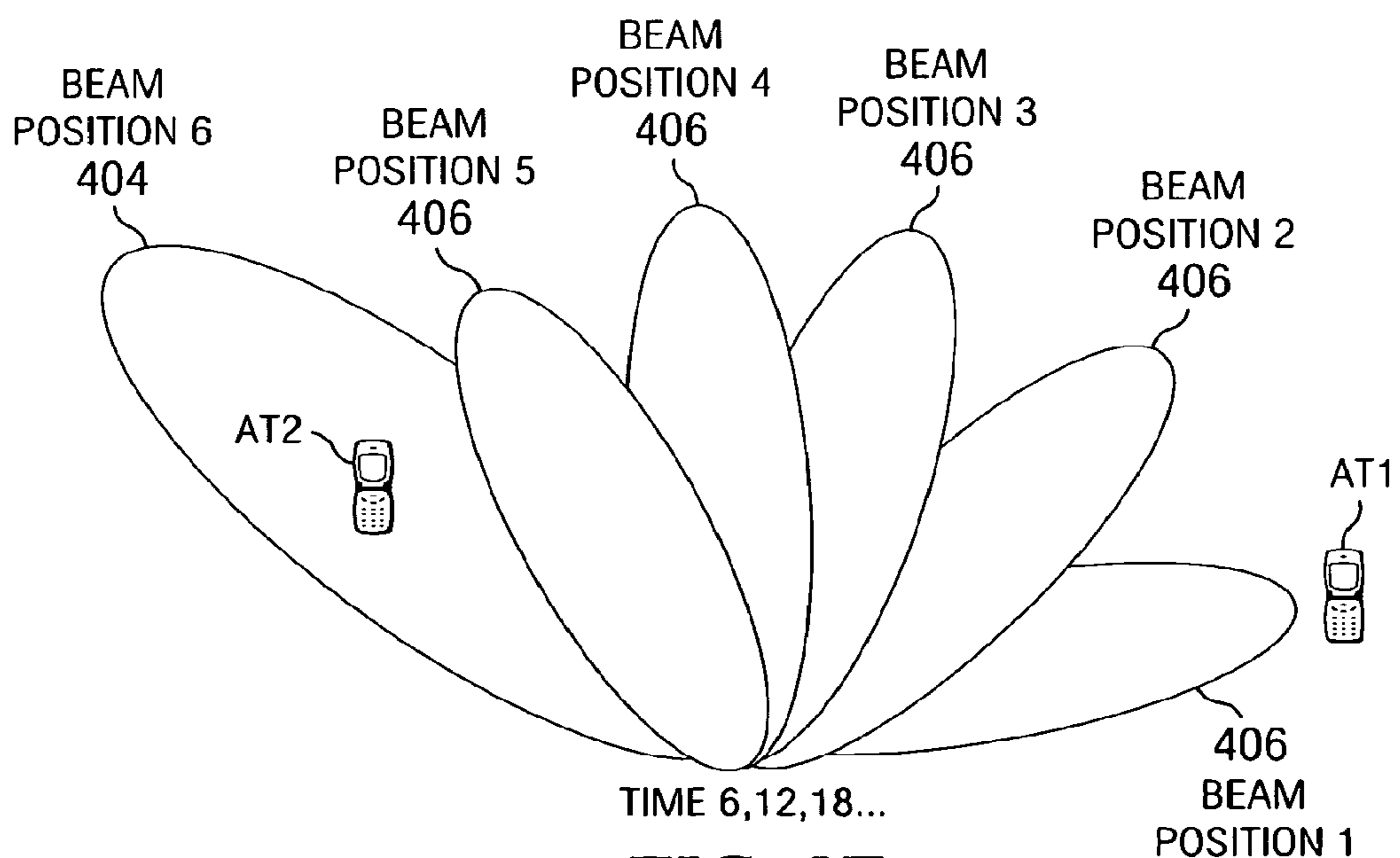
FIG. 5F
