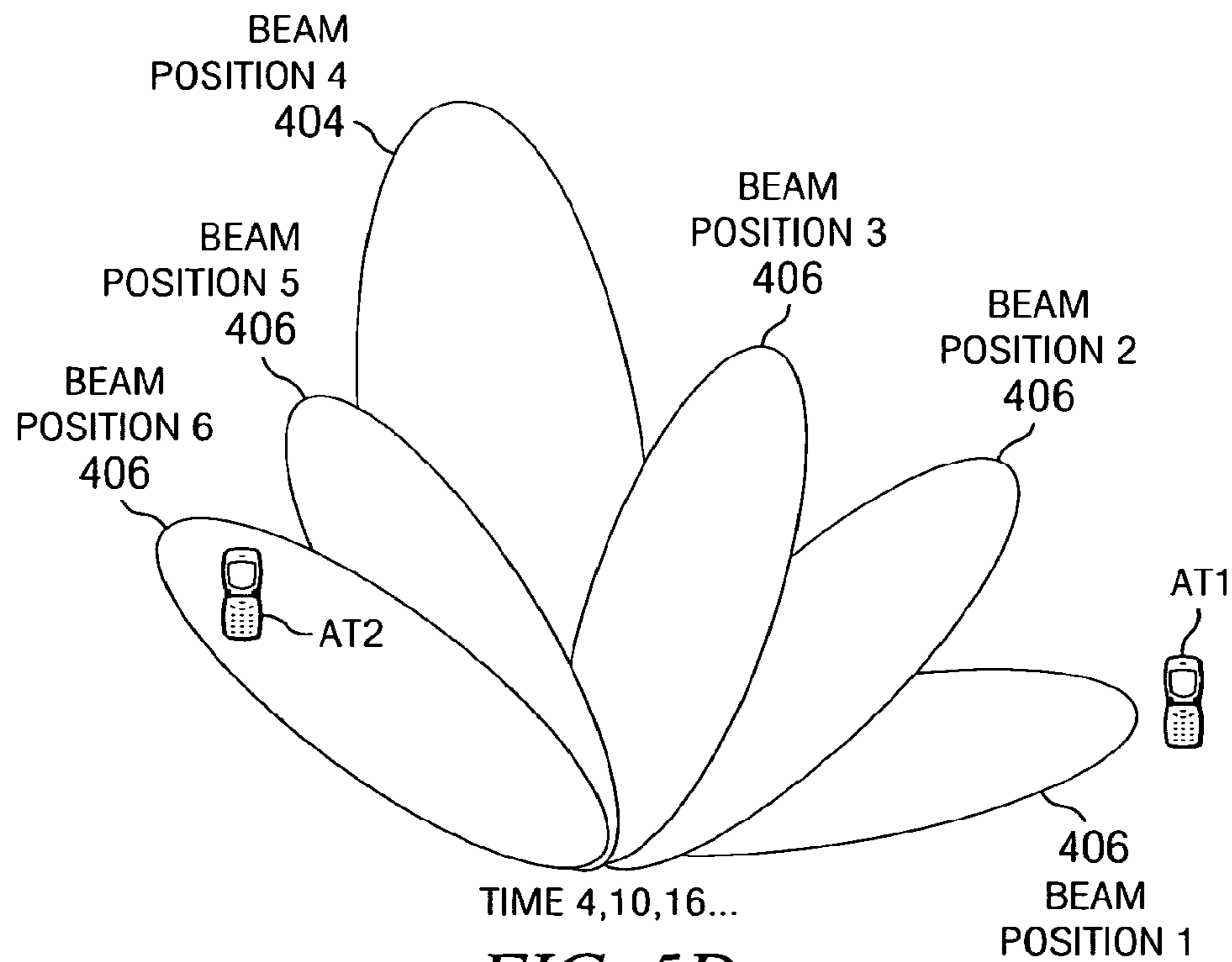
FIG. 5D
