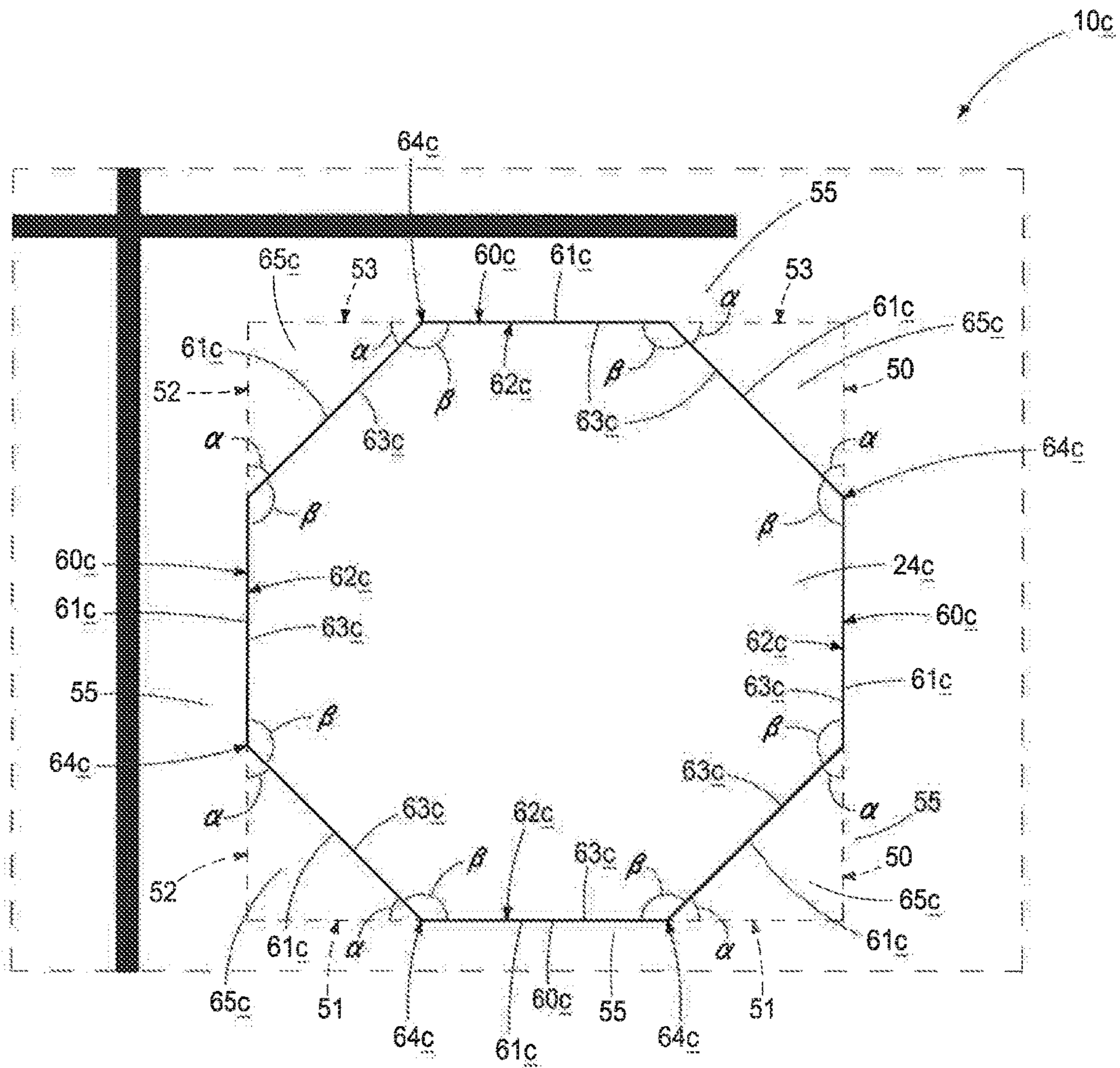
FIG. 6A
