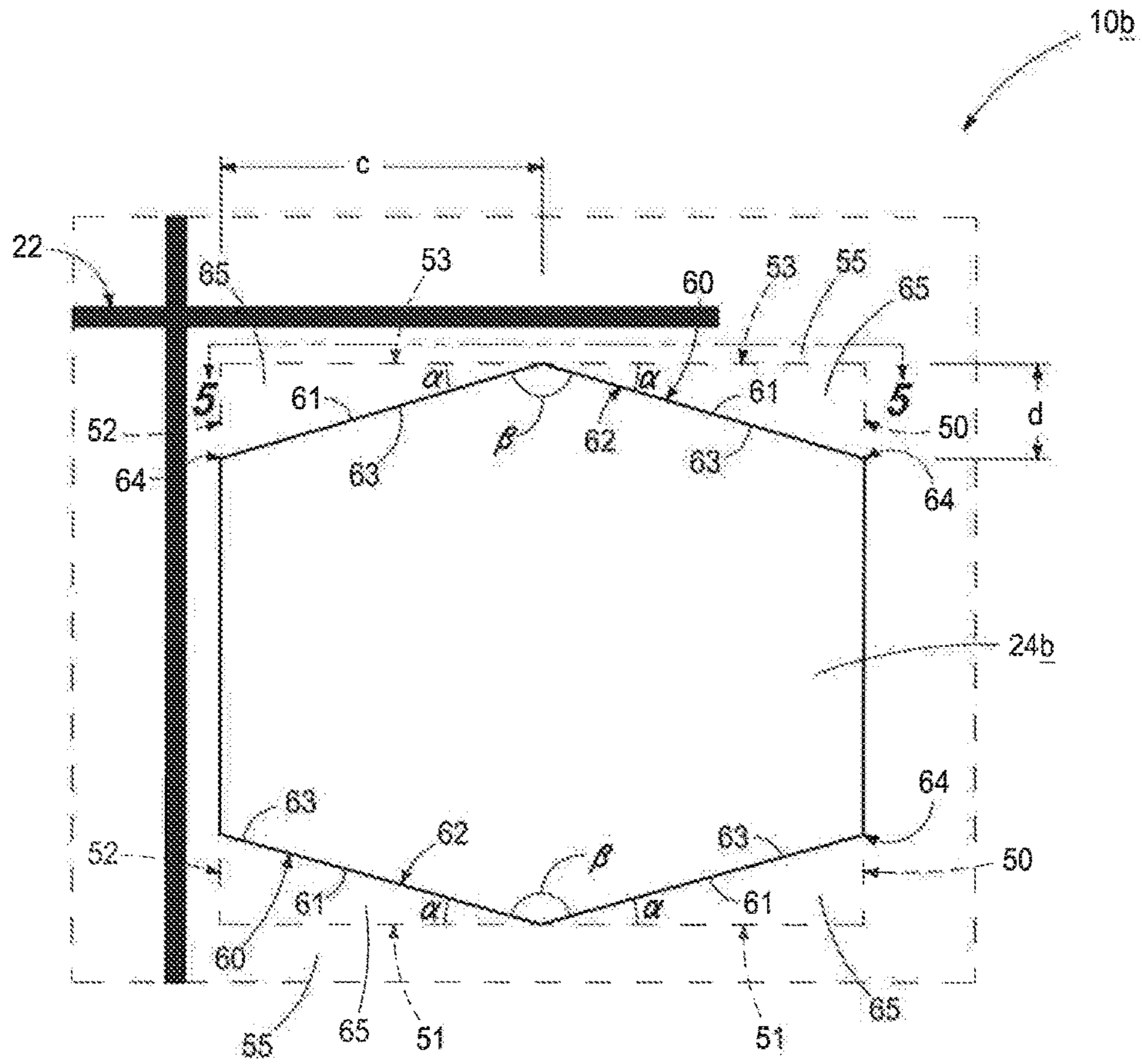
FIG. 4A
