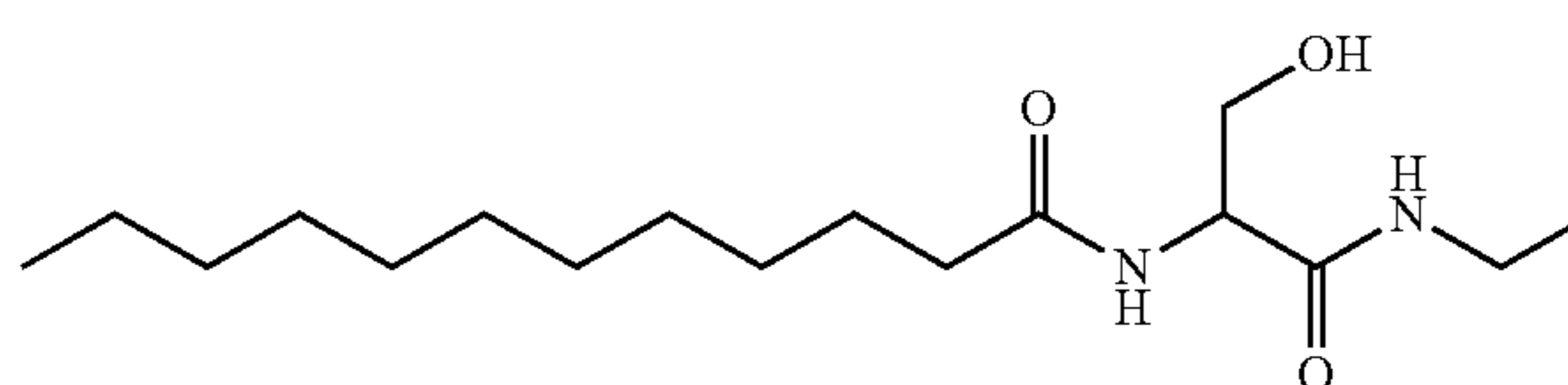
N-(1-((ethylamino)-3-hydroxy-1-oxopropan-2-yl)dodecanamide
