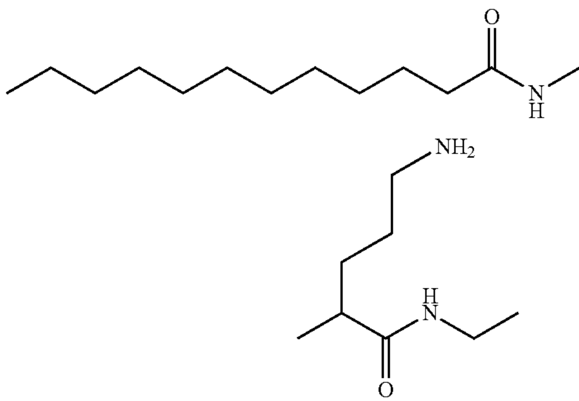
N-(4-amino-1-(ethylcarbamoyl)butyl)dodecanamide;
