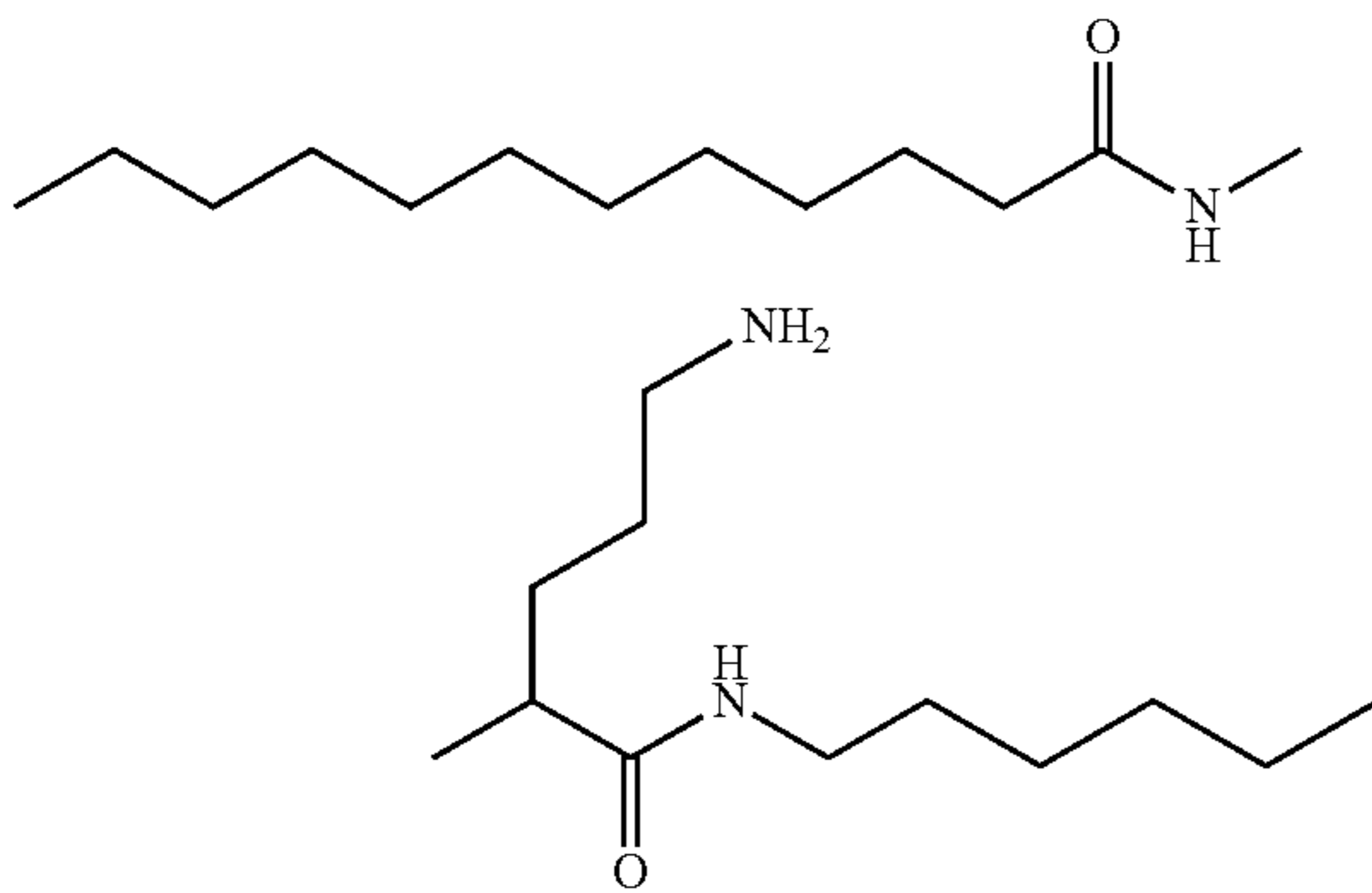
N-(4-amino-1-(ethylcarbamoyl)butyl)dodecanamide;
