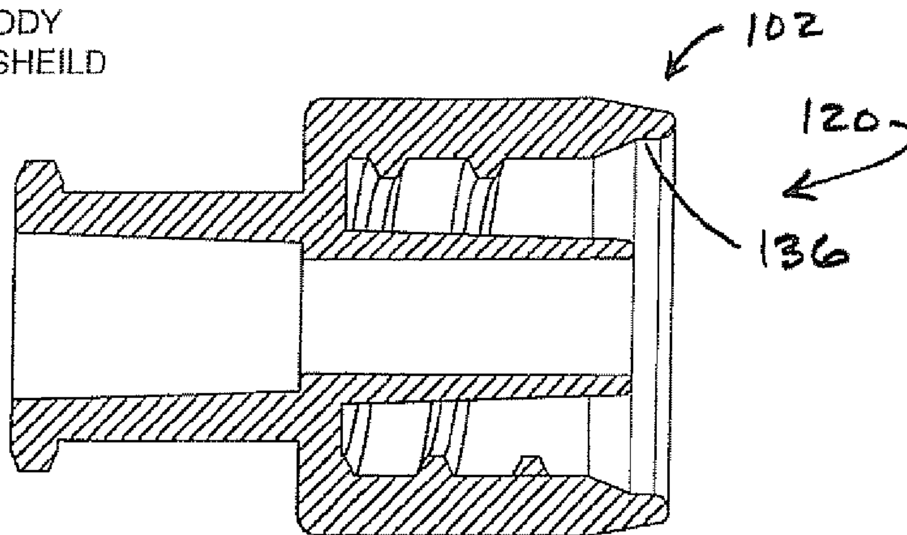
SECTION A-A
