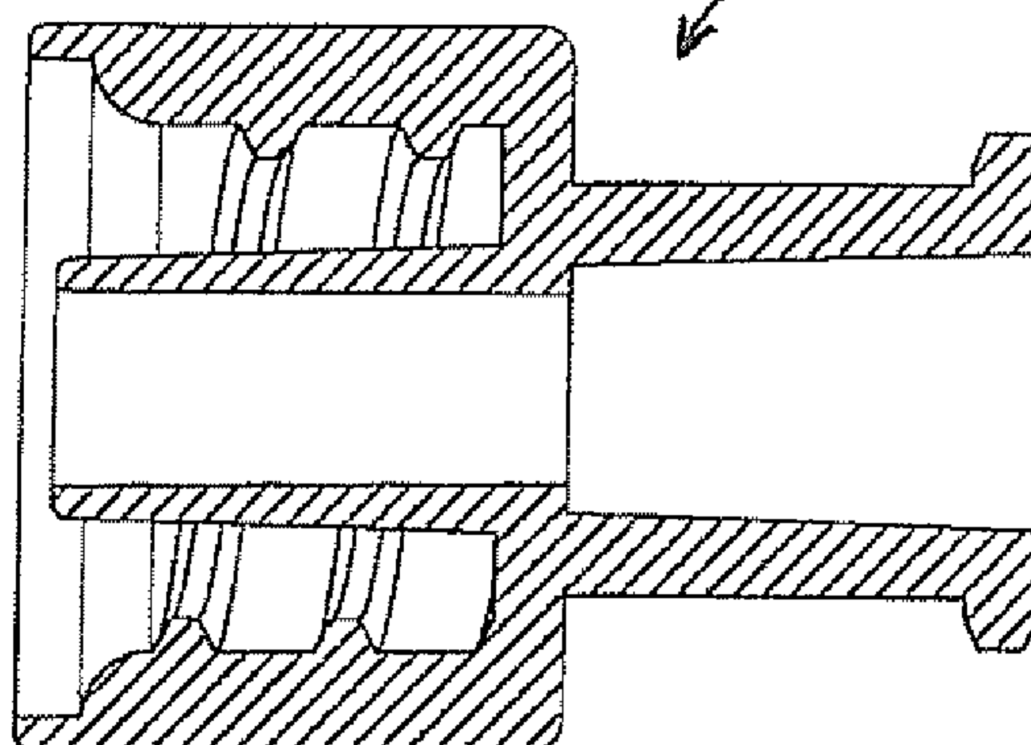
SECTION A-A
