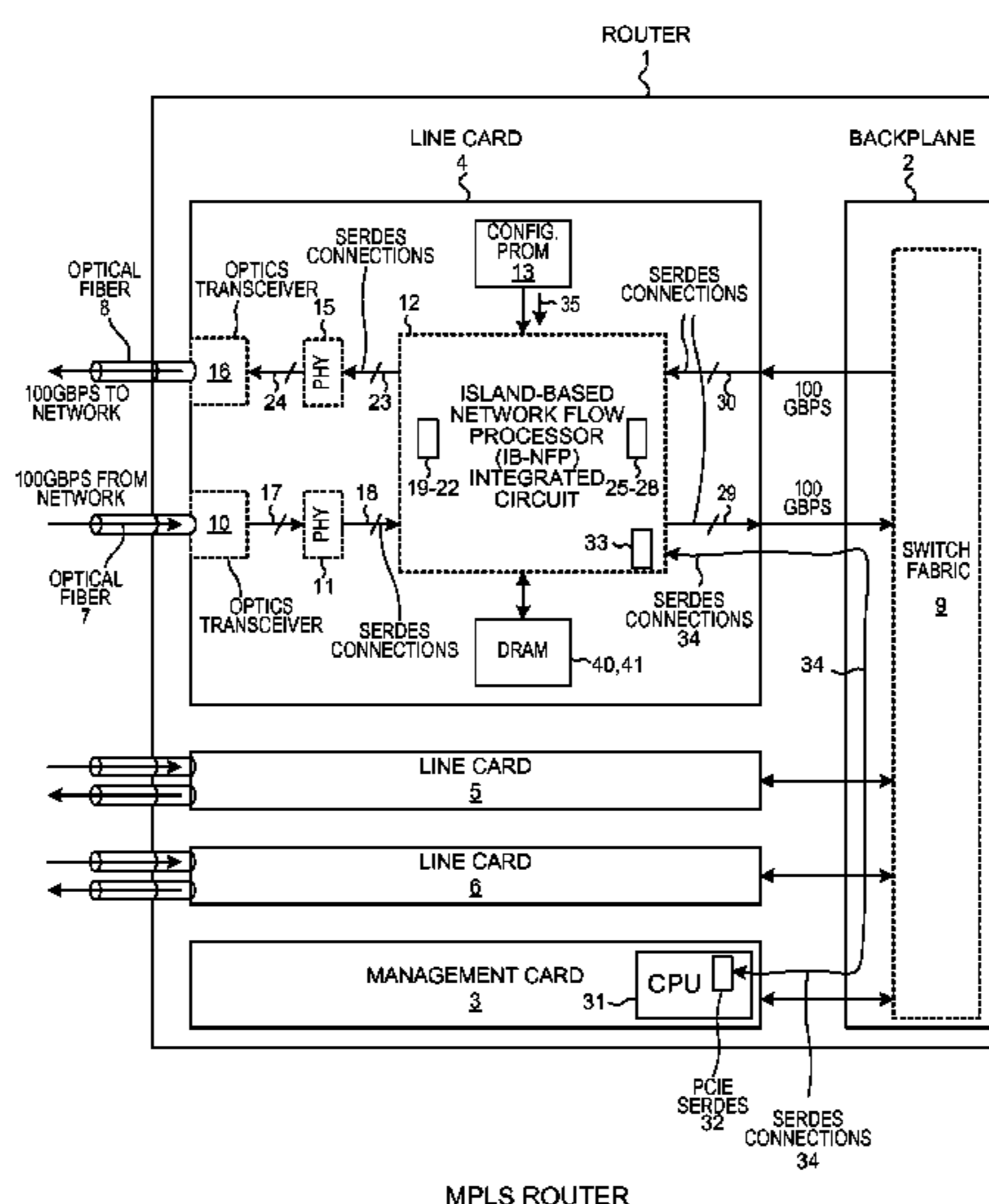
MPLS ROUTER
