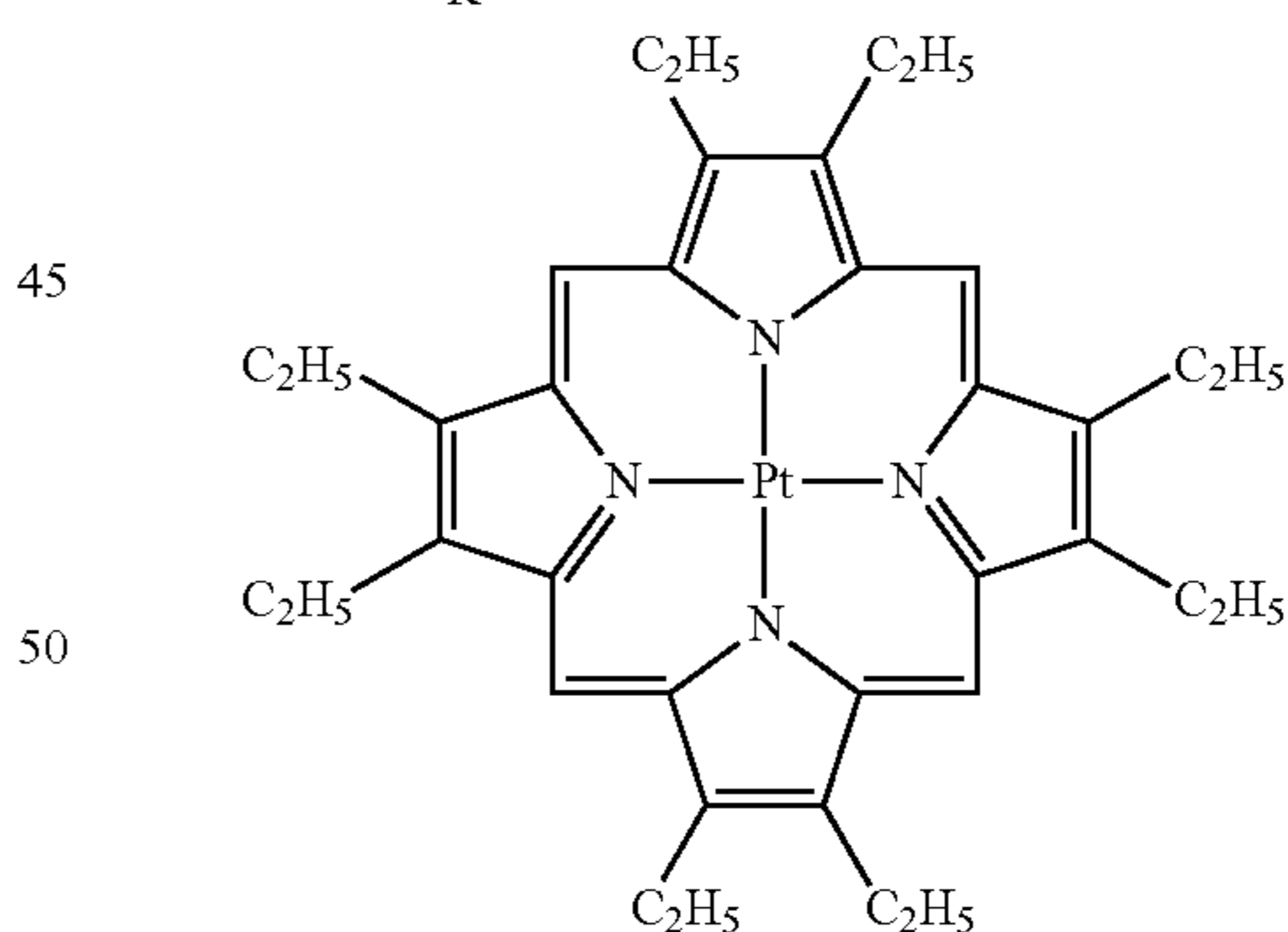
PtOEP
