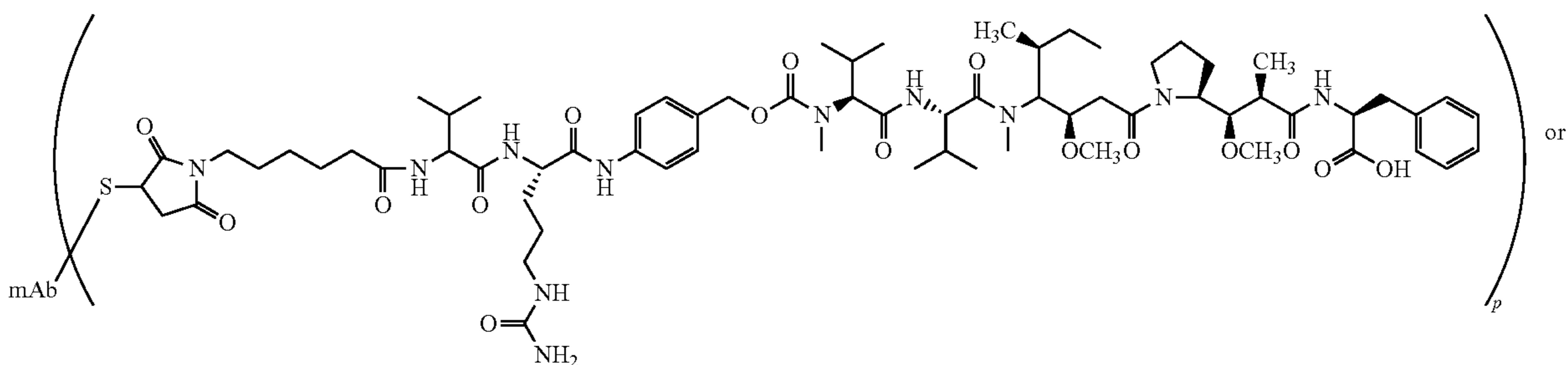
L-MC-vc-PAB-MMAE.
