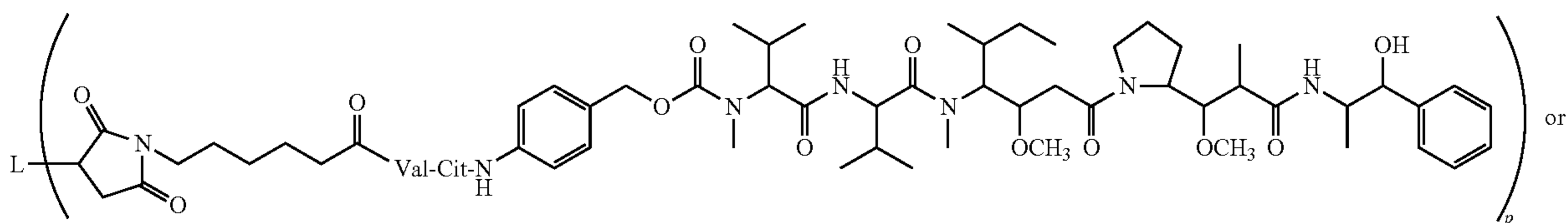
L-MC-vc-PAB-MMAF
