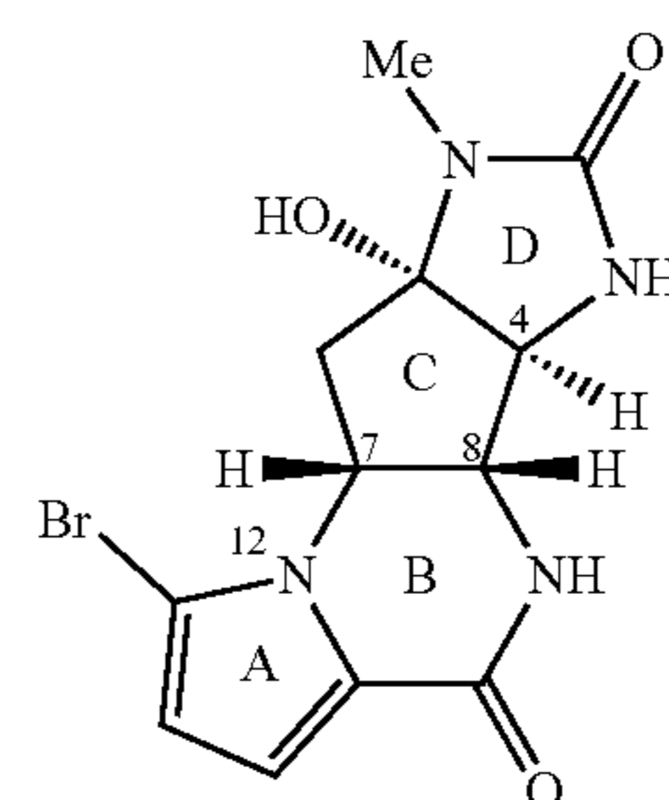
(-)-agelastatin A
