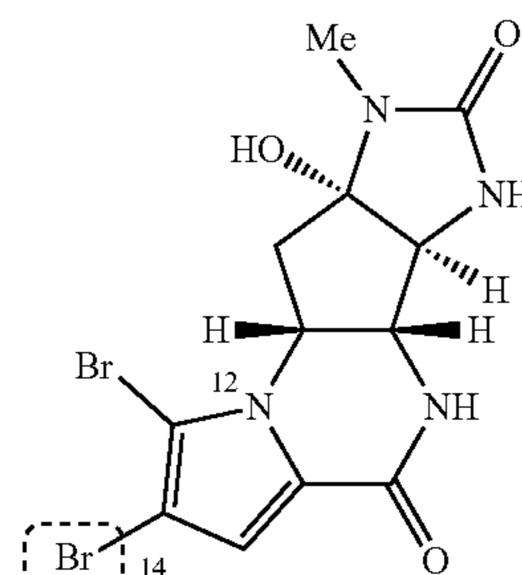
(-)-agelastatin B
