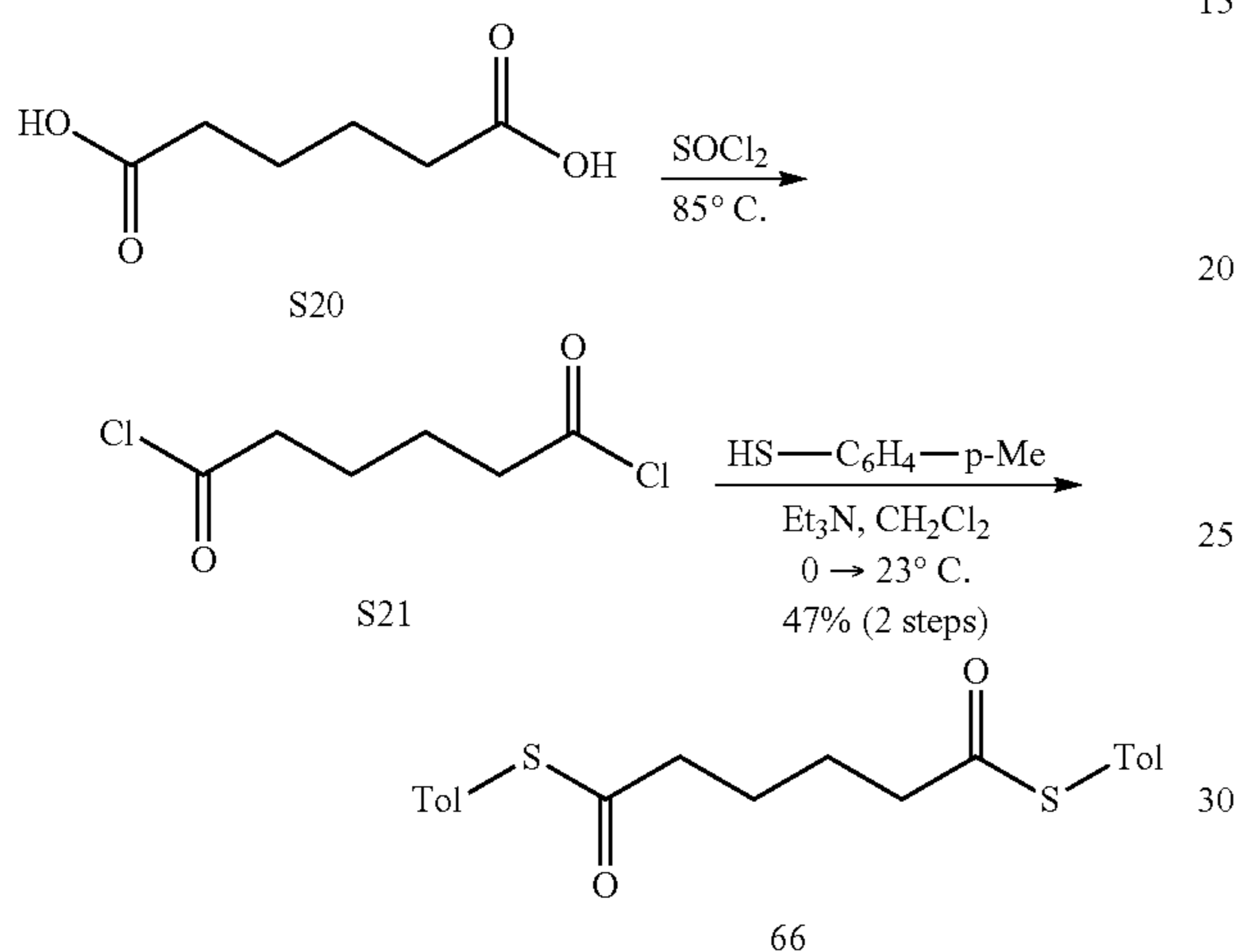
S,S-Di-p-tolyl hexanebis(thioate) 66
