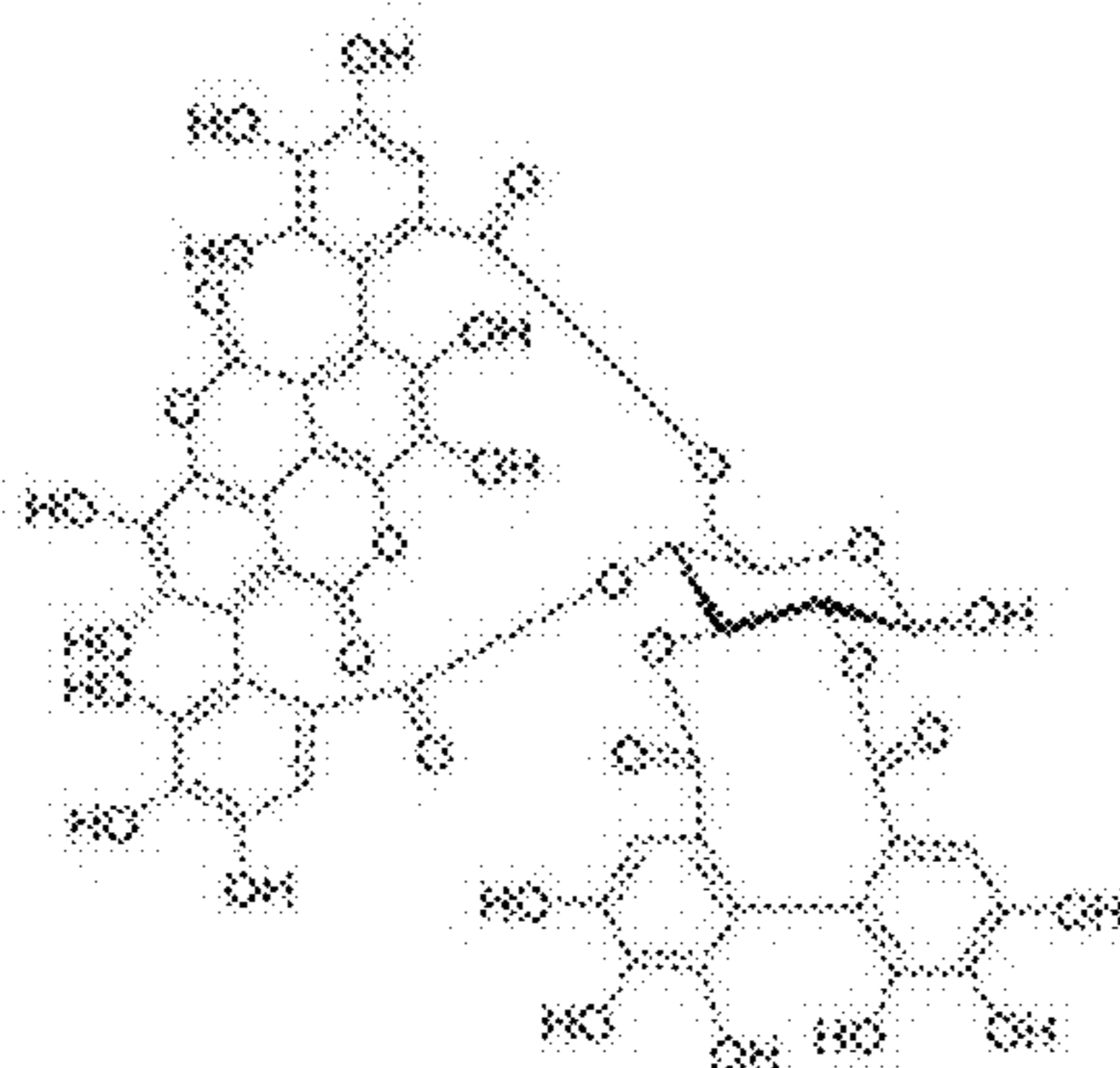
Punicalagin (PA)
