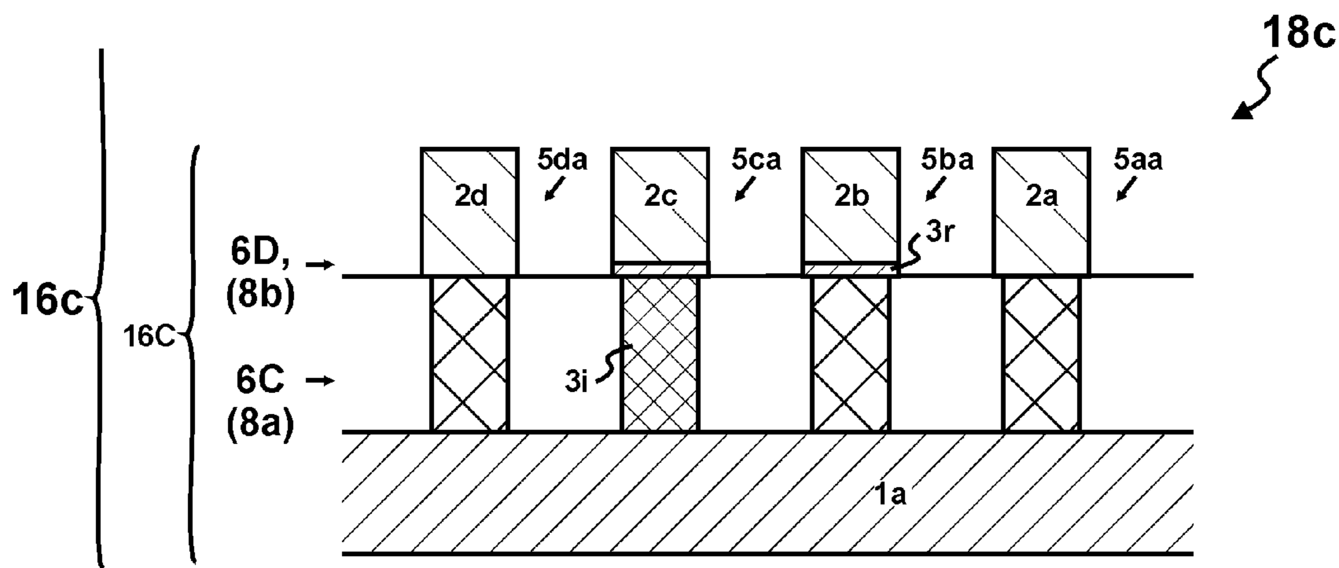
Fig. 10A
