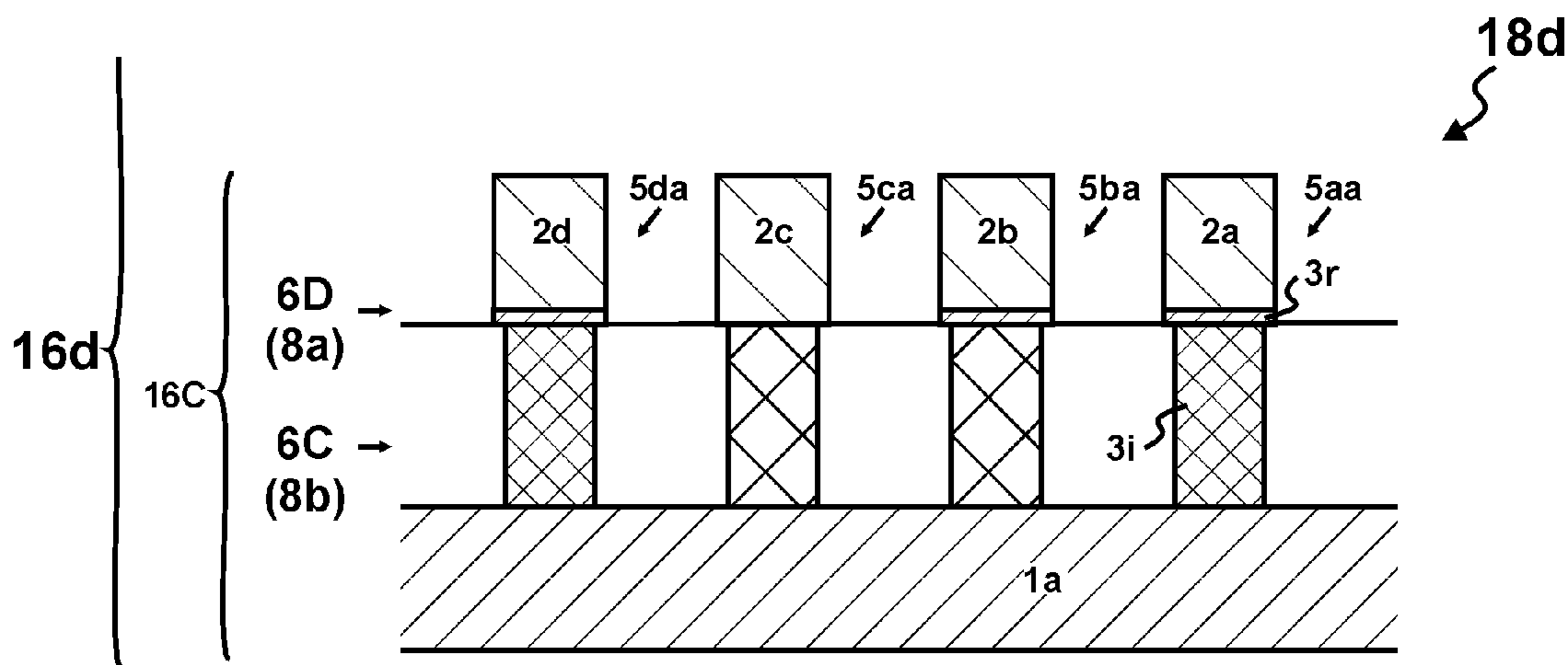
Fig. 10B
