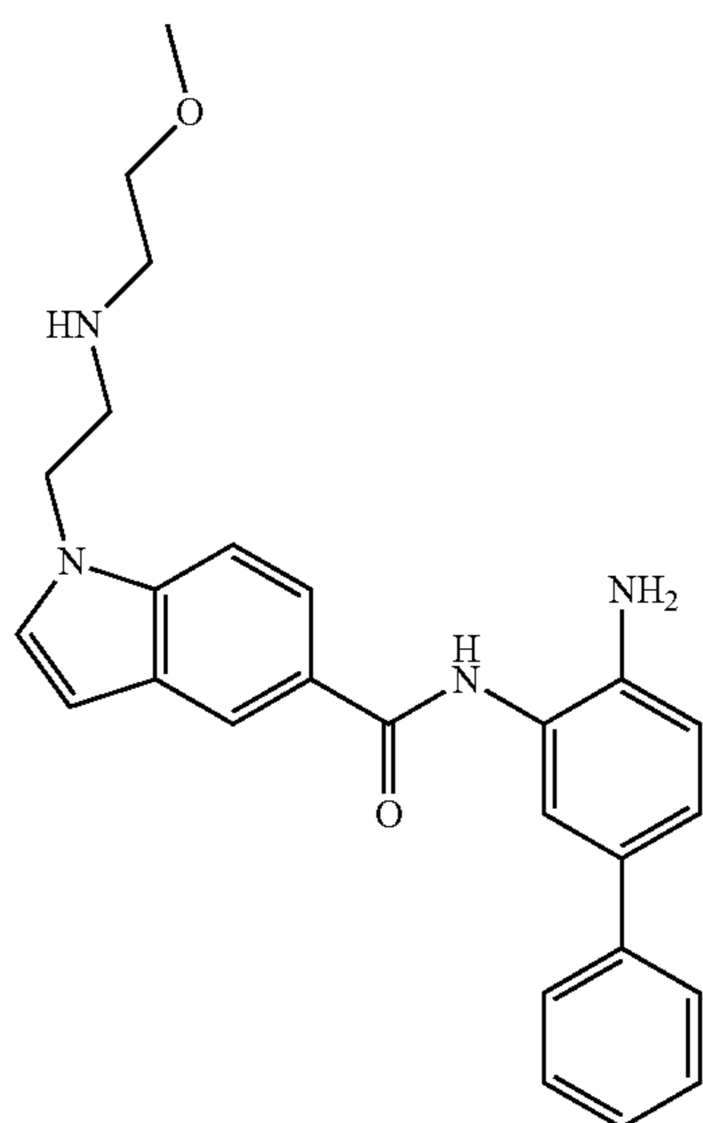
N-(4-amino-[1,1'-biphenyl]-3-yl)-1-(2-((2-methoxyethyl)amino)ethyl)-1H-indole-5-carboxamide
