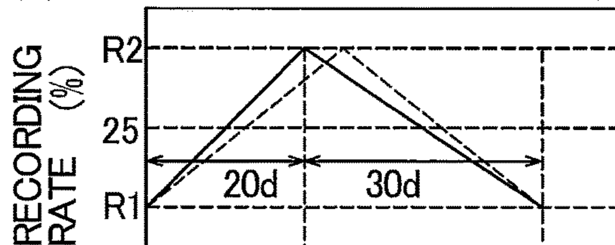
(D) GRADED RECORDING RATE DR (9)
